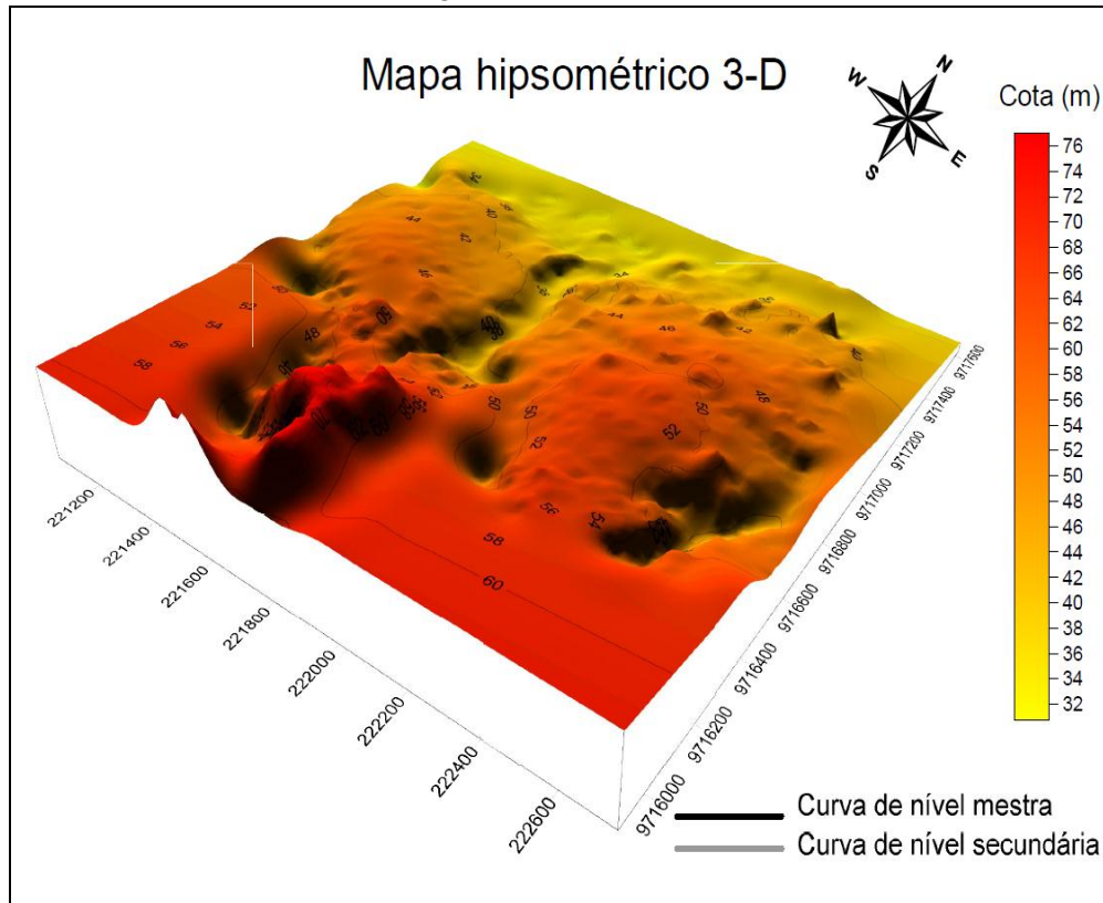
Figura 5: Modelo 3-D.
