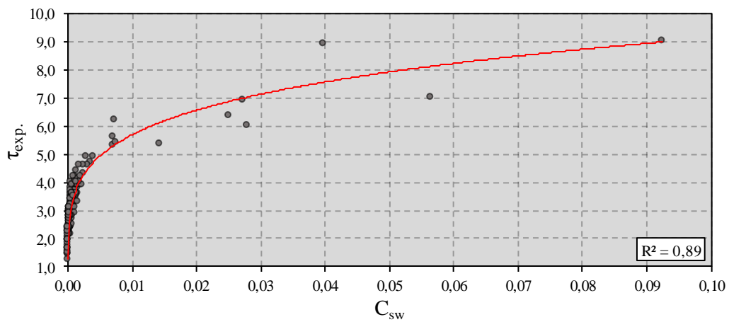
Figura 3.5 – Correlação entre tensão última e C_{sw}
