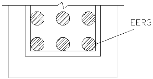
Figura 3.19 - Posicionamento dos extensômetros na armadura de flexão
