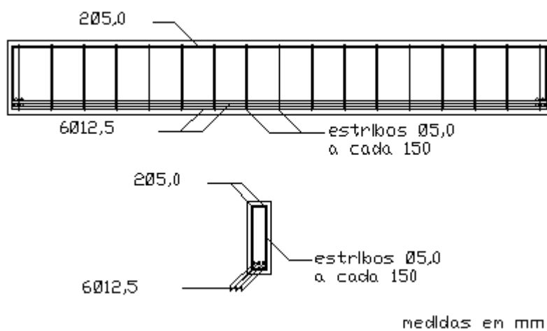
Figura 3.13 - Detalhe da armadura da viga VPF6
