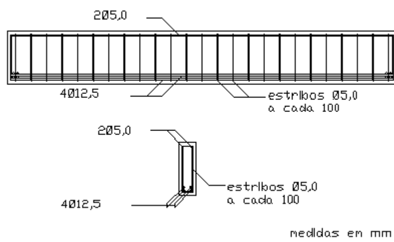
Figura 3.9 - Detalhe da armadura da viga VPF2
