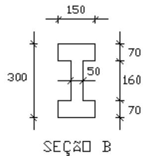
Figura 2.34 - Vista lateral e seções das vigas (LEITE JÚNIOR, 2000)
