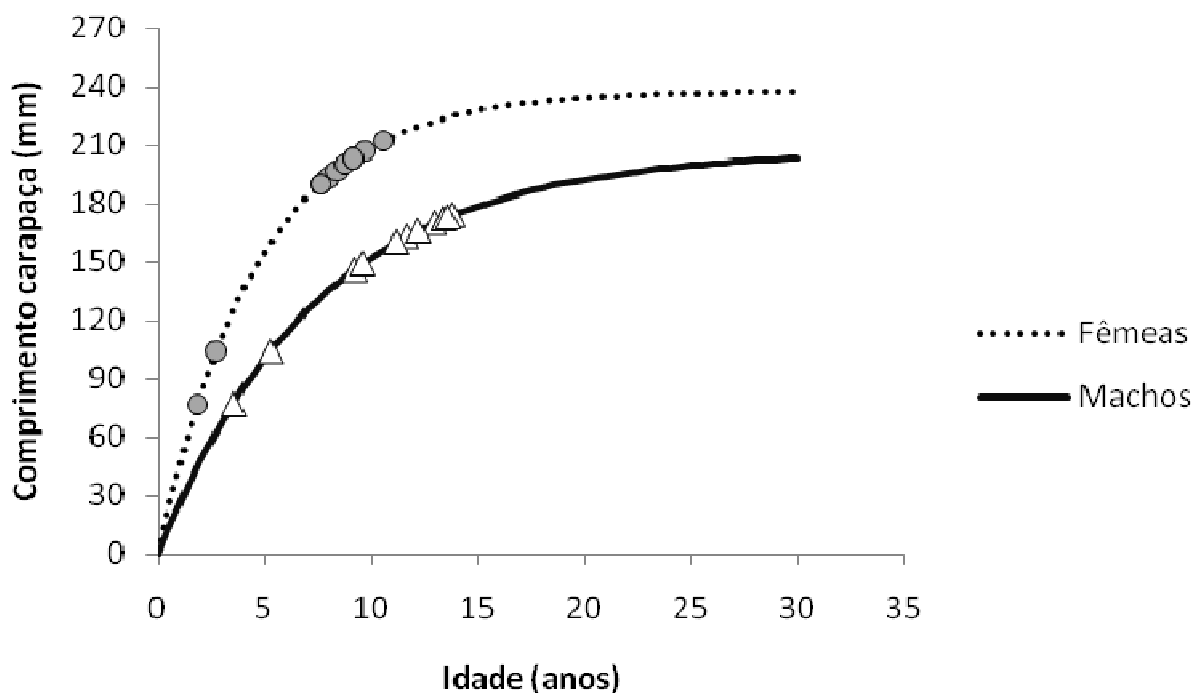
Figura 13: Curva de crescimento ajustada ao modelo de von Bertalanffy, baseada nos valores de K e L_{\infty} estimados pelo método de Gulland e Holt (1959), para as fêmeas e os machos de R. p. punctularia . Os círculos indicam as fêmeas e os triângulos os machos que foram capturados e recapturados na APA de Algodal/Maiandeuá, Maracanã, Pará.
