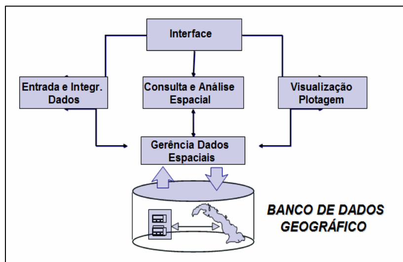
Figura 3: Visão Geral de um SIG
