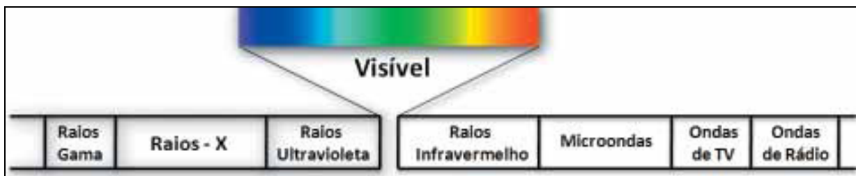
Figura 1: Espectro eletromagnético, com destaque para a região do visível.
