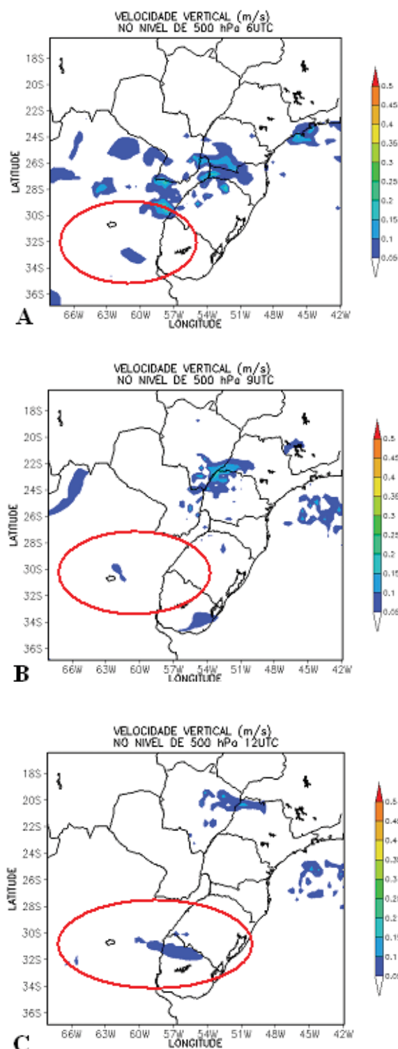
Figura 6 Velocidade Vertical (ms-1) simulada pelo modelo BRAMS em 500 hPa para o dia 27/11/2002. (A) 06:00 UTC - fase de iniciação, (B) 09:00 UTC - fase de maturação e (C) 12:00 UTC - fase de dissipação. O círculo mostra a região do CCM.
