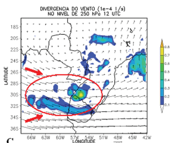
Figura 5 Vento ( ms^{-1} ) e Divergência ( 10^{-4}\ s^{-1} ) simulados pelo modelo BRAMS em 250 hPa para o dia 27/11/2002. (A) 06:00 UTC - fase de iniciação, (B) 09:00 UTC - fase de maturação e (C) 12:00 UTC - fase de dissipação. As setas mostram o JAN e o círculo a região do CCM.
