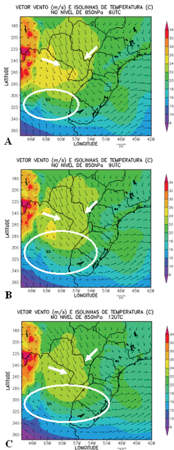
Figura 3 Vento (ms -1 ) e isolinhas de temperatura (°C) simulados pelo modelo BRAMS em 850 hPa para o dia 27/11/2002. (A) 06:00 UTC - fase de iniciação, (B) 09:00 UTC - fase de maturação e (C) 12:00 UTC - fase de dissipação. As setas mostram o JBN e o círculo a região do CCM.
