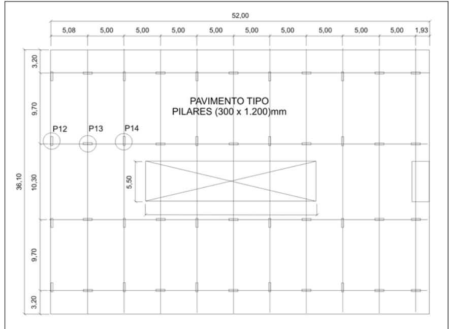
Figura 4 - Disposição dos pilares no pavimento tipo.
