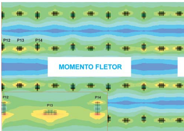
Figura 5 - Contorno dos momentos-fletores nas lajes.
