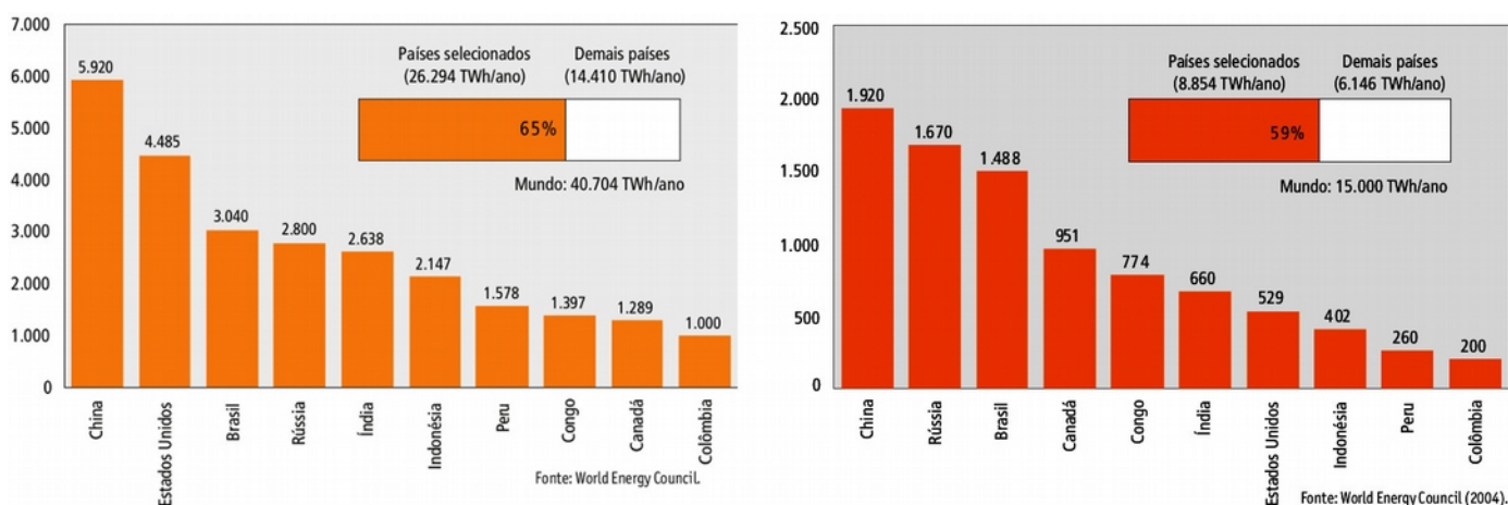
Figura 3 - Potencial hidrelétrico teórico no mundo e Potencial Hidrelétrico Tecnicamente aproveitável no mundo em Twh/ano.
