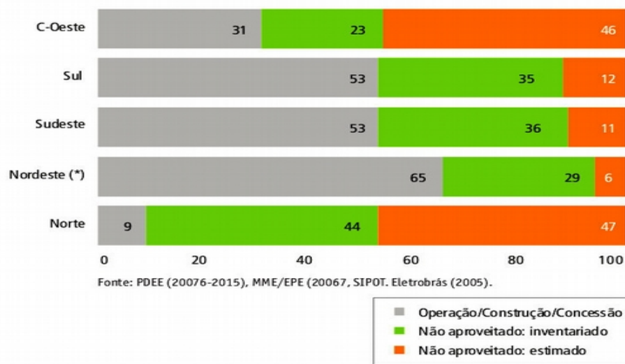
Figura 4 - Aproveitamento do Potencial Hidrelétrico Brasileiro, por região %.
