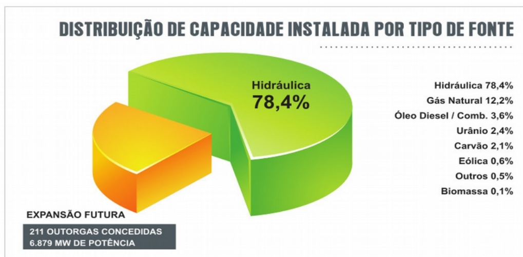
Figura 2 - Distribuição da capacidade instalada por tipo de fonte.
