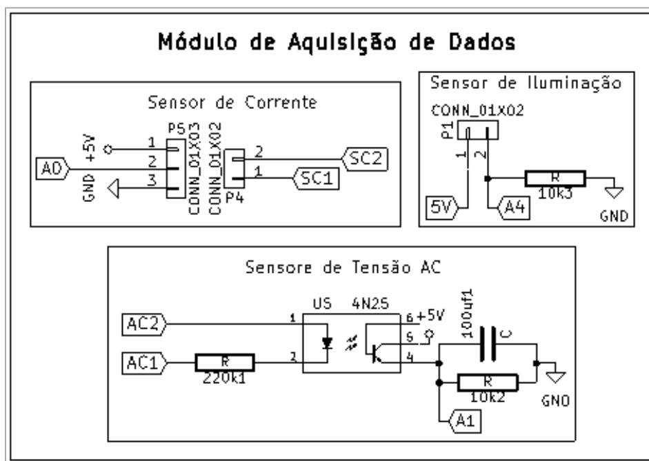
Figura 5.4 – Diagrama estrutural do nó de medição para iluminação residencial.
