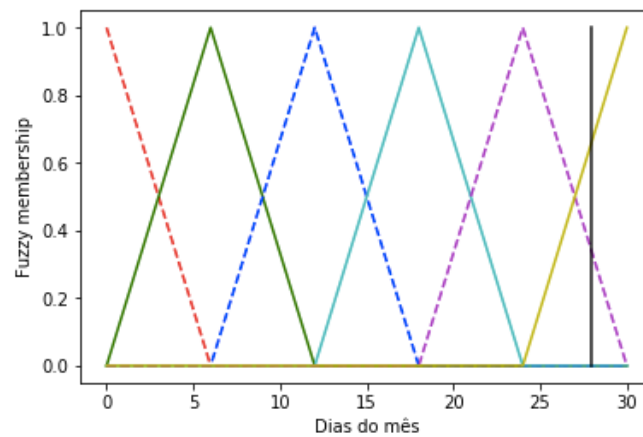
Figura 6.20 - Entrada “% do mês” no sistema Fuzzy.
