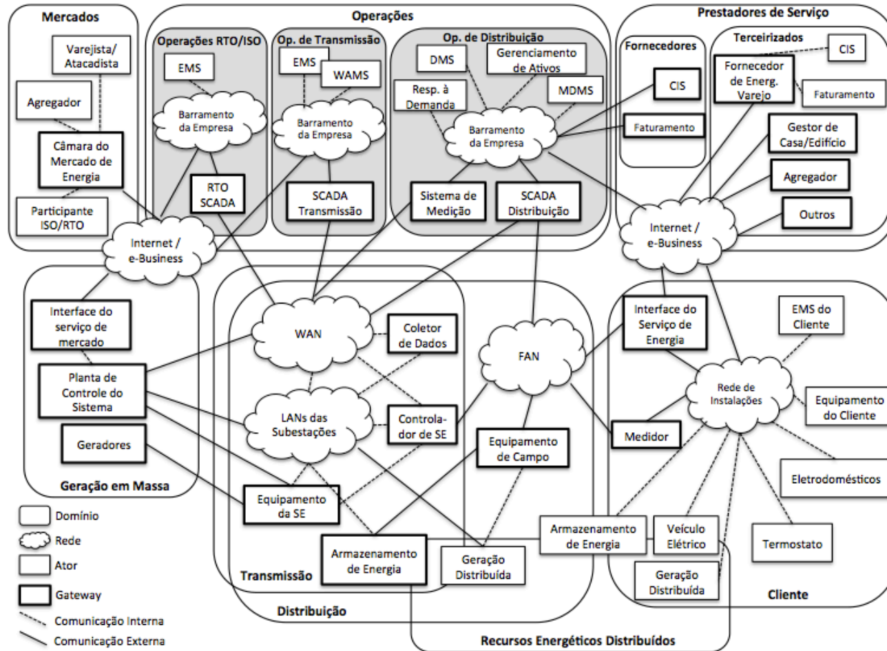
Figura 2.2 – Diagrama conceitual de referência para a rede de transmissão de dados do Smart Grid .
