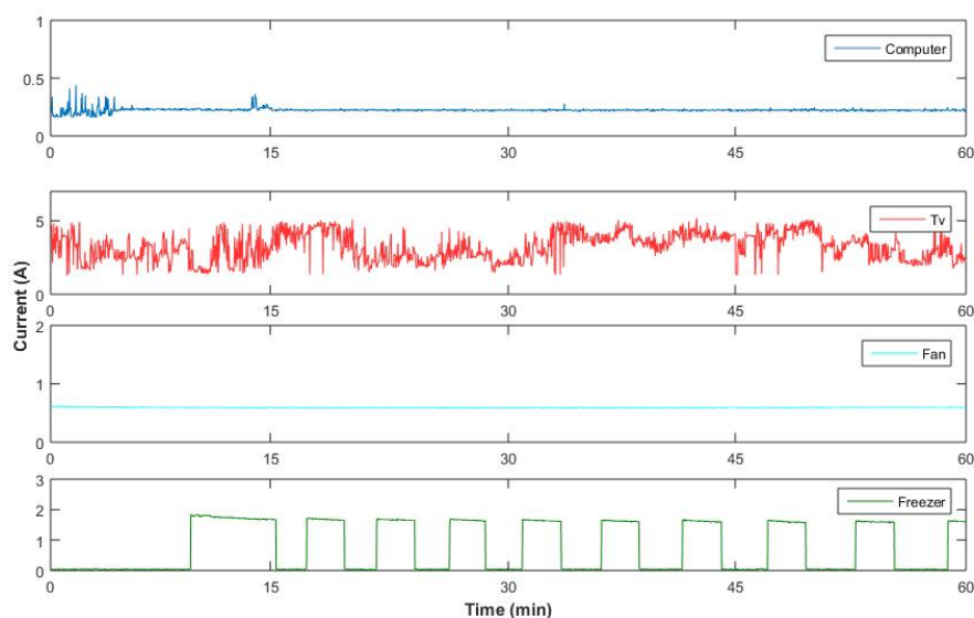
Figura 6.4 – Visualização da corrente
