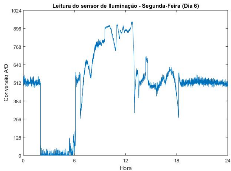
Figura 6.12 - Monitoramento de iluminação (Dia 6).
