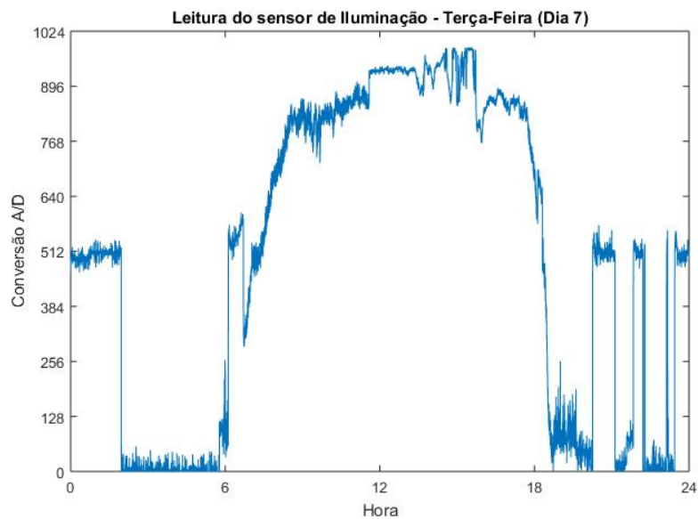
Figura 6.13 - Monitoramento de iluminação (Dia 7).
