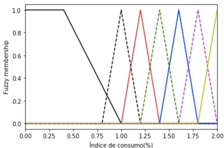
Figura 6.16 - Entrada “Índice de Consumo” no sistema Fuzzy.
