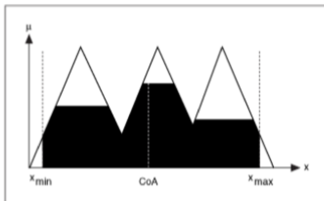
Figura 3.4 - Defuzzificação tipo Centro de Área.
