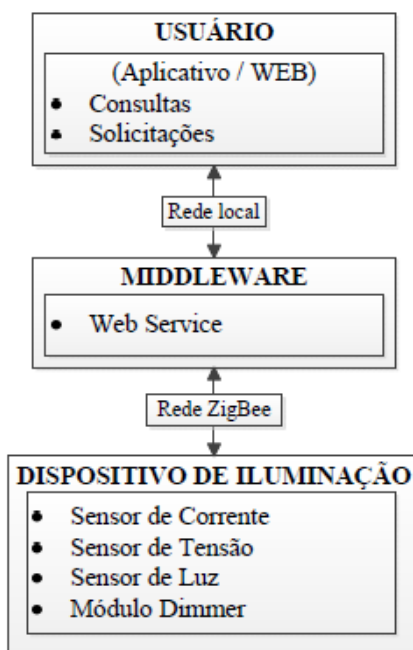
Figura 6.6 – Diagrama conceitual do modelo de gerenciamento de iluminação.
