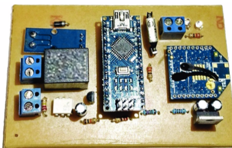
Figura 5.5 – Protótipo do nó de medição
