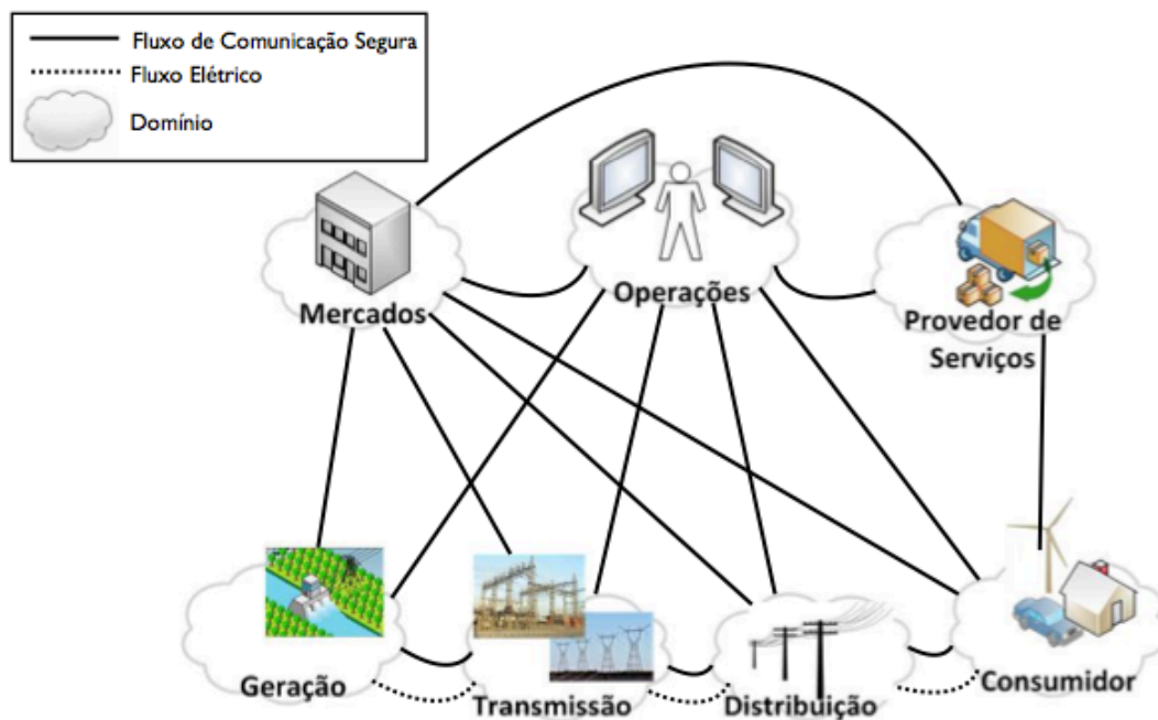
Figura 2.1 –Interação entre os atores de diferentes domínios.
