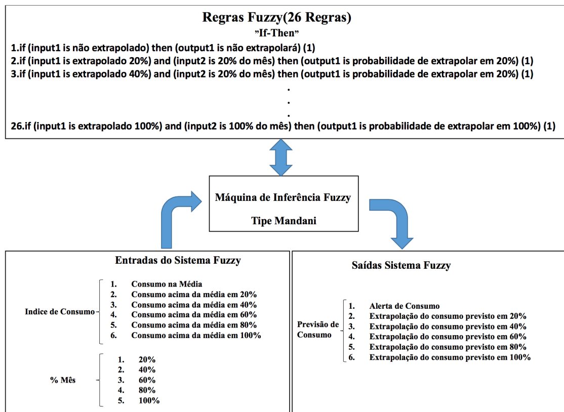
Figura 6.15 - Overview do sistema Fuzzy.
