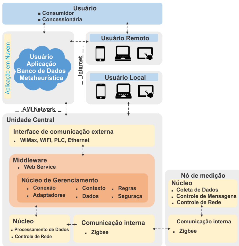
Figura 5.2 – Diagrama da Arquitetura Smart CoM
