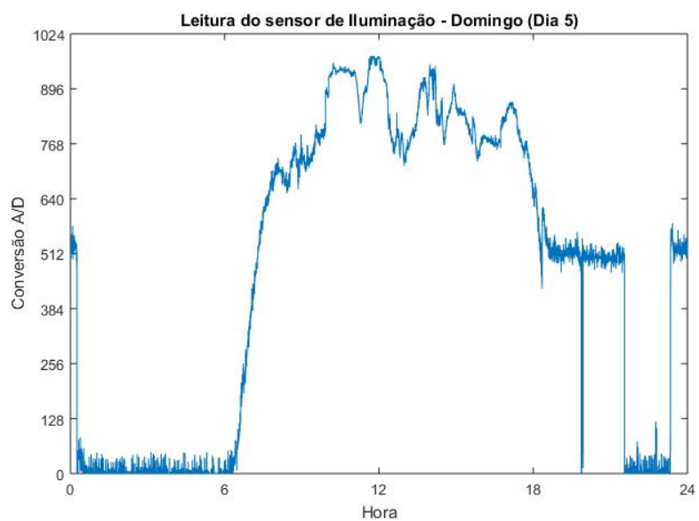
Figura 6.11 - Monitoramento de iluminação (Dia 5)
