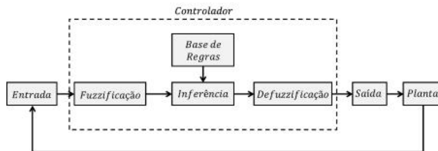
Figura 3.3 - Estrutura básica de um sistema de controle Fuzzy.
