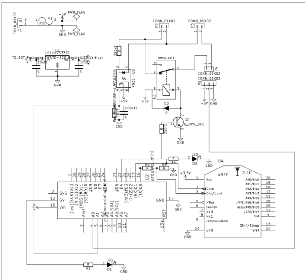
Figura 5.3 – Diagrama estrutural do nó de medição
