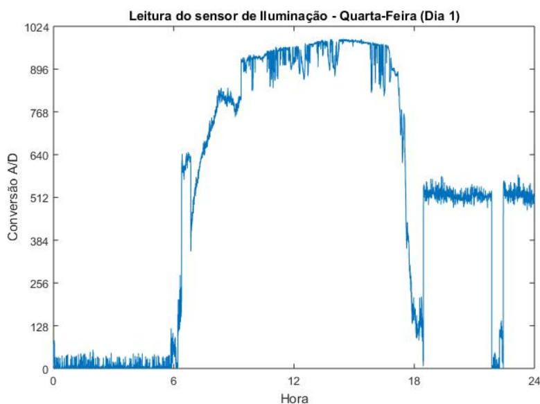
Figura 6.7 - Monitoramento de iluminação (Dia 1)
