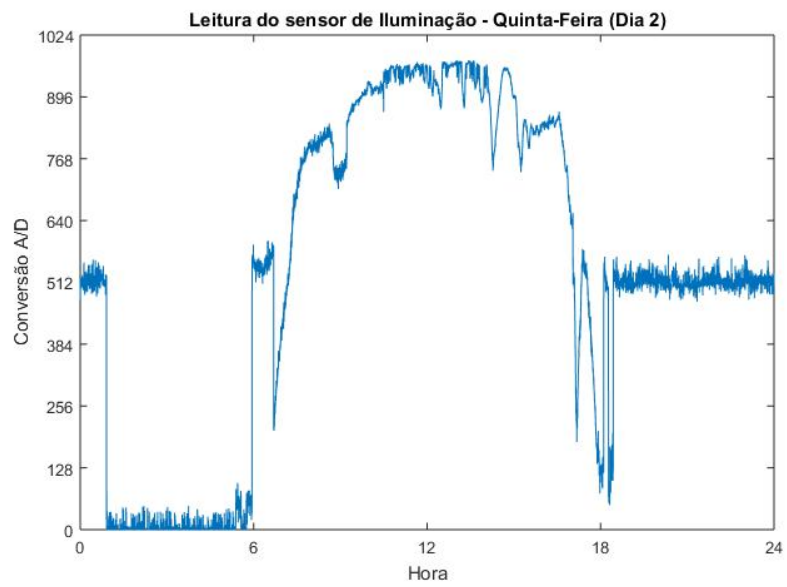
Figura 6.8 - Monitoramento de iluminação (Dia 2)
