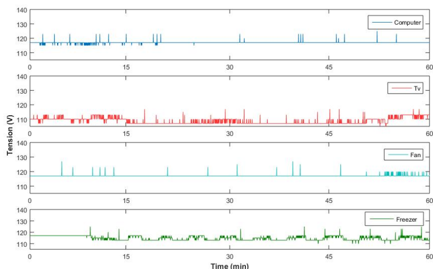
Figura 6.5 – Visualização da tensão.
