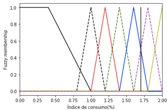
Figura 6.21 - Entrada “Índice de consumo” no sistema Fuzzy.
