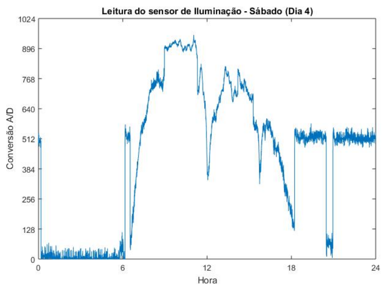
Figura 6.10 - Monitoramento de iluminação (Dia 4).
