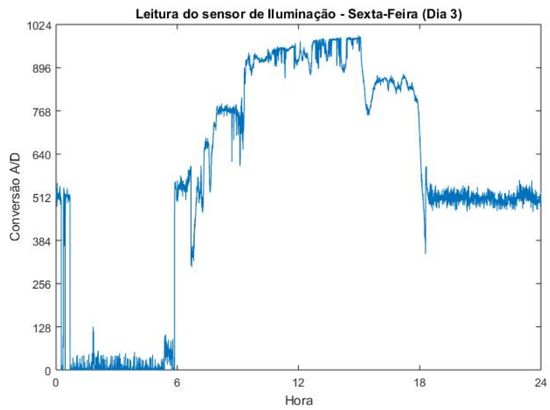
Figura 6.9 - Monitoramento de iluminação (Dia 3).
