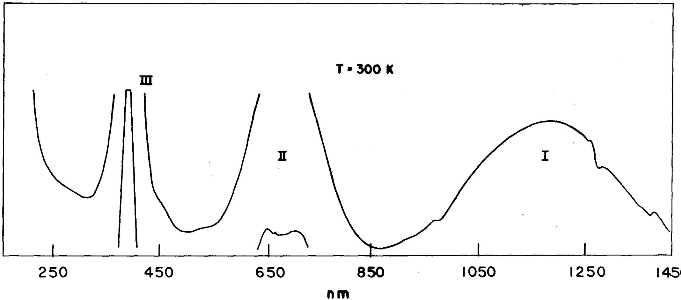
FIG III.5 - Espectro de absorção do \alpha SNH a temperatura ambiente.
