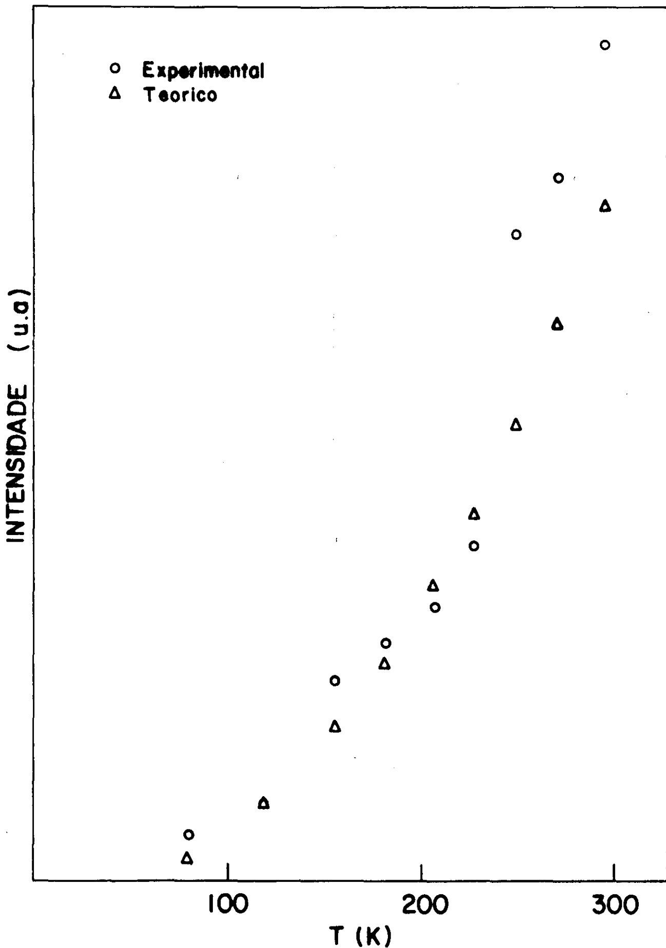
FIG IV.8 Dependência com a temperatura da intensidade da linha A anti stokes comparada com o processo de diferença de dois fonons.
