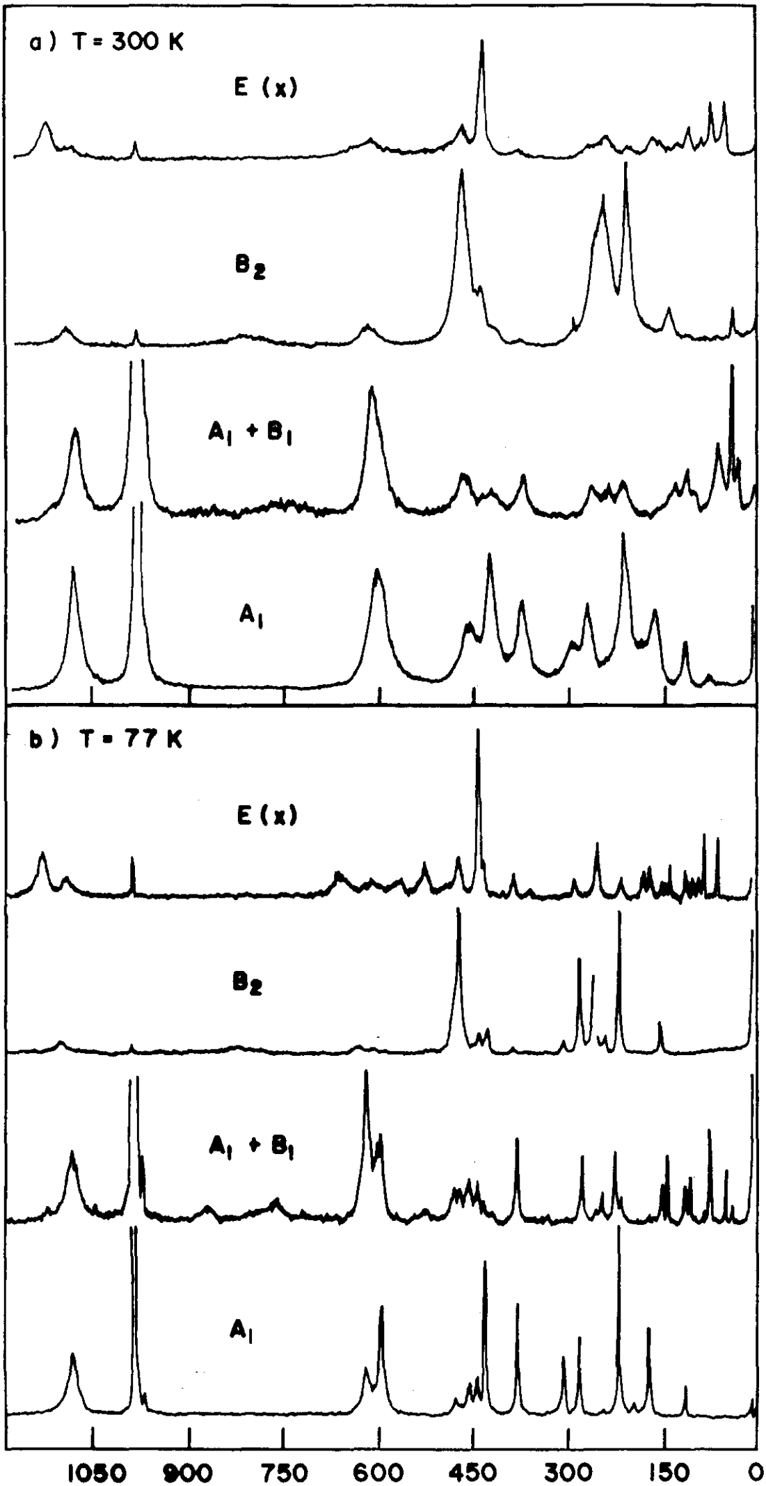
FIG III. B - ESPECTRO RAMAN DO MONOCRISTAL \text{NiSO}_4 \cdot 6\text{H}_2\text{O} (Região de 0 a 1200\text{ cm}^{-1} )
