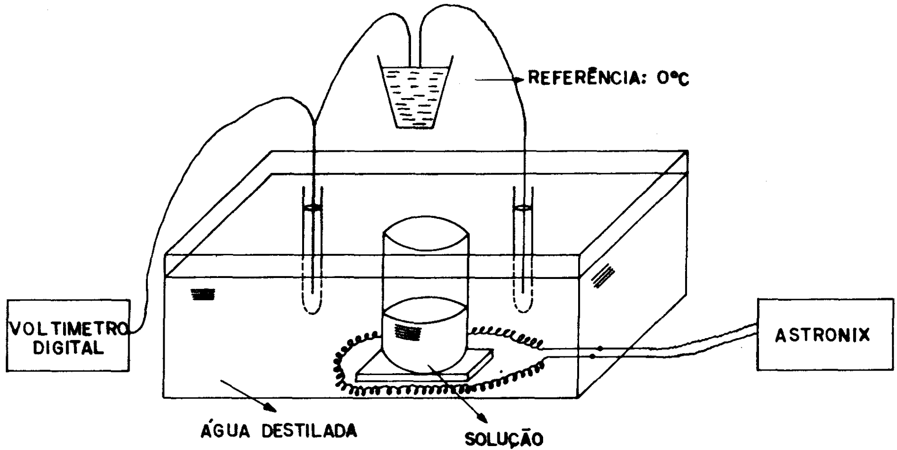
FIG III.1 - Montagem experimental para crescimento das amostras.
