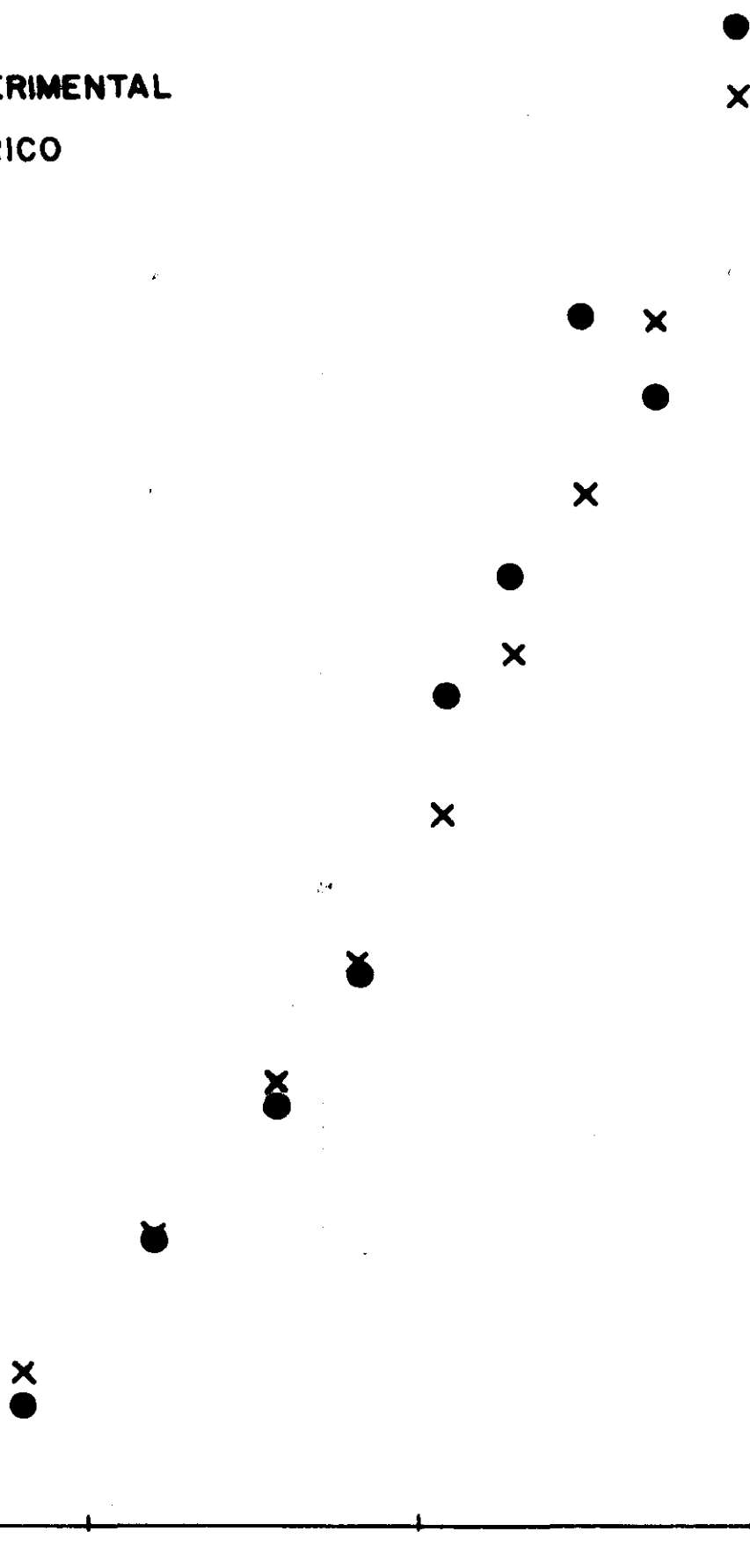
FIG IV.7 - Dependência com a temperatura da intensidade da linha A stokes comparada com o processo de diferença de dois fonons.
