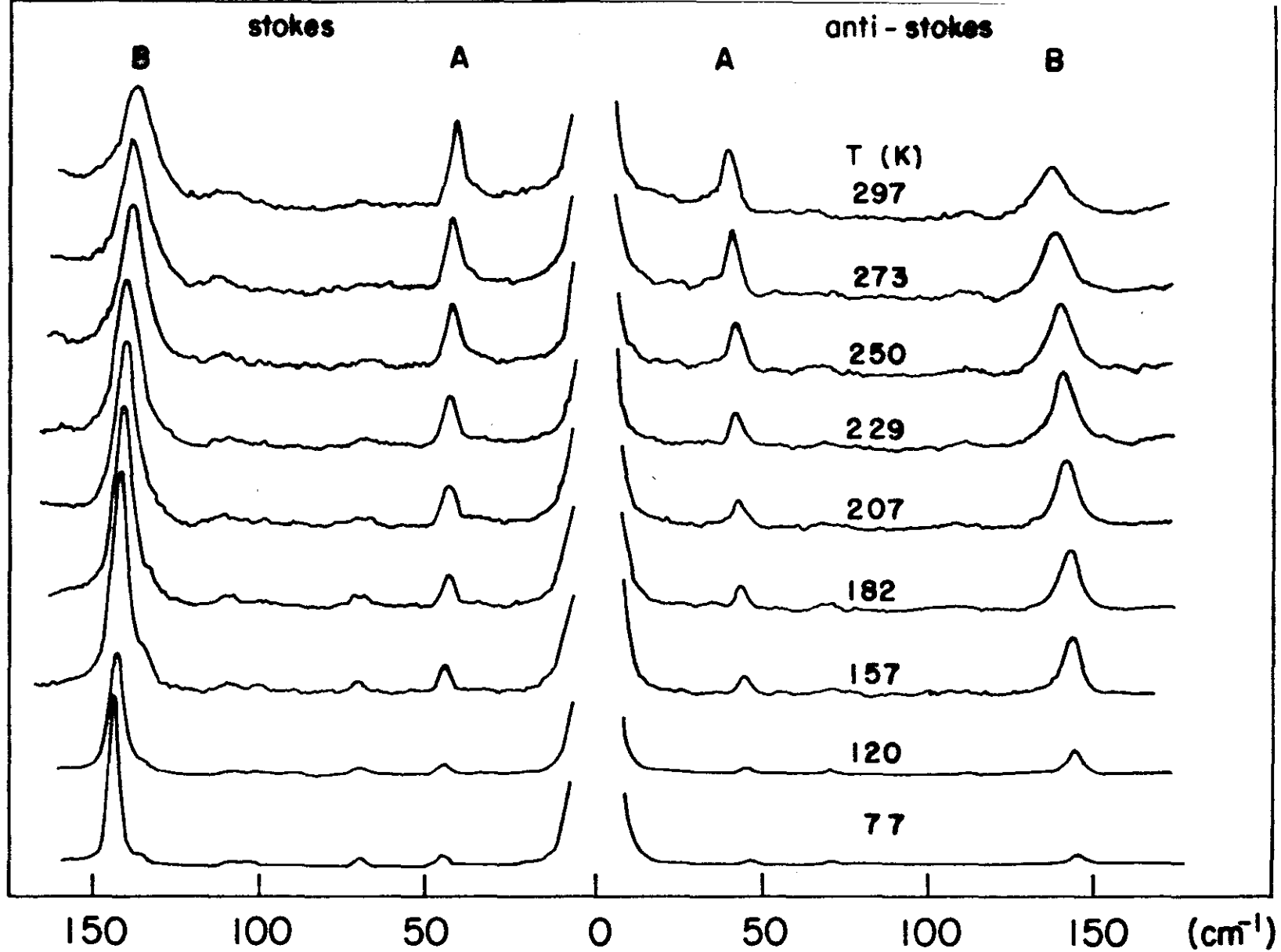
FIG IV. 4 - Comportamento das linhas A e B em função da temperatura
