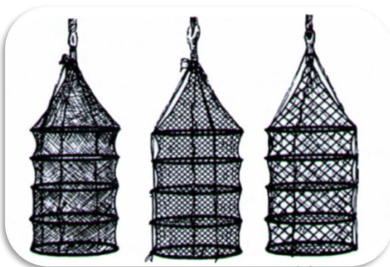
Figura 6 Lanternas de cultivo (Alcântara Neto, 2003).
