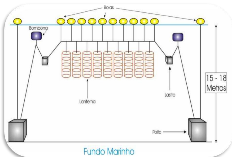
Figura 4 Esquema de instalação de espinhel para cultivo de ostra. Foto: Leonardo Zayas Fonseca.
