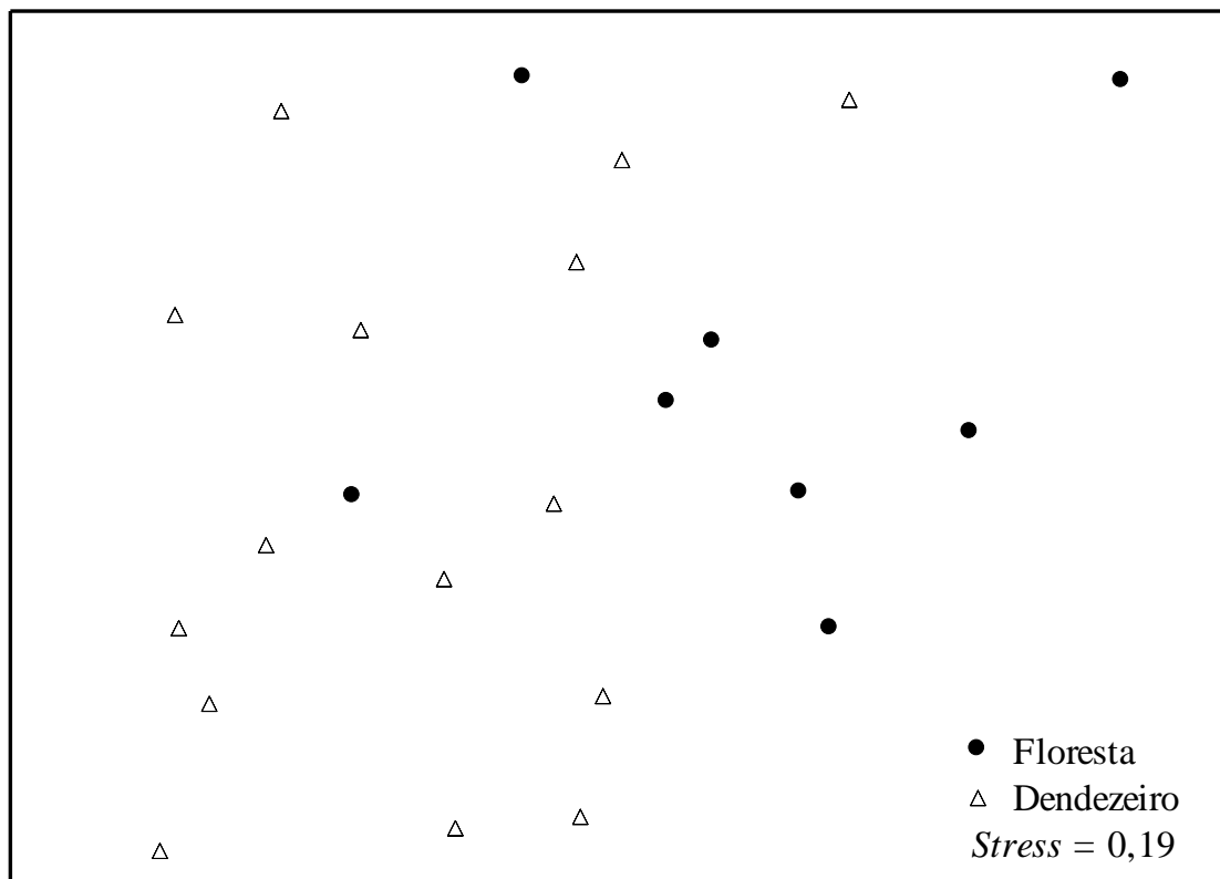
399 400 Figura 4 - Ordenamento produzido pelo escalonamento multidimensional não métrico 401 baseado na abundância e composição das espécies de peixes dos igarapés amostrados 402 em áreas de fragmentos florestais e áreas de monocultura de dendezeiro na Amazônia 403 Oriental, Nordeste do Estado do Pará, Norte do Brasil.
