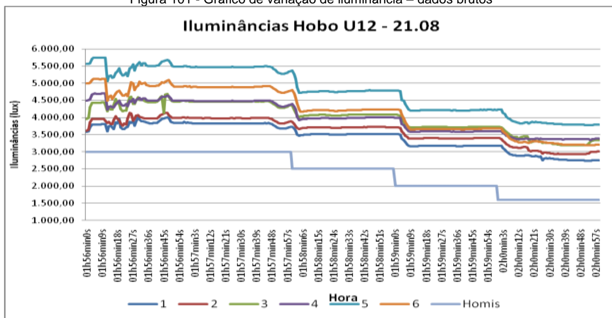
Figura 101 - Gráfico de variação de iluminância – dados brutos
