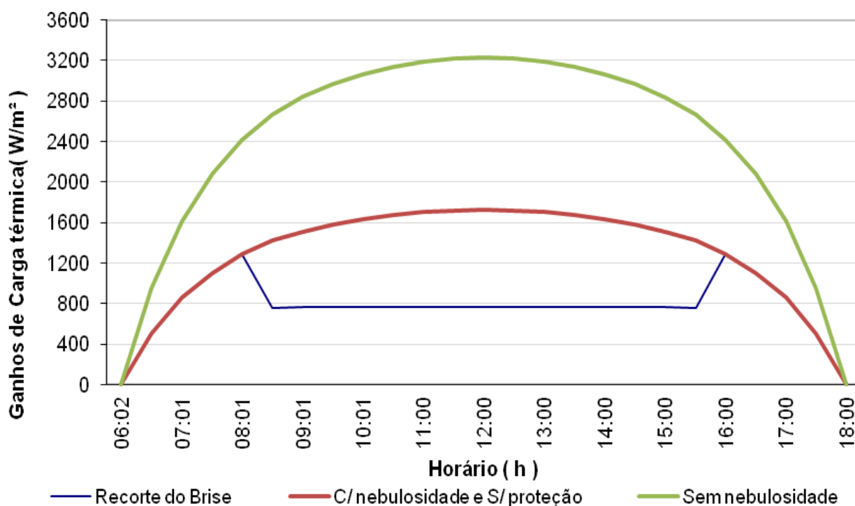
Figura 56 - Variação horária dos ganhos totais de calor solar para a fachada norte, dia 22 de junho e Nebulosidade 6.1 – dados obtidos do programa Arqitrop e luz do sol.
