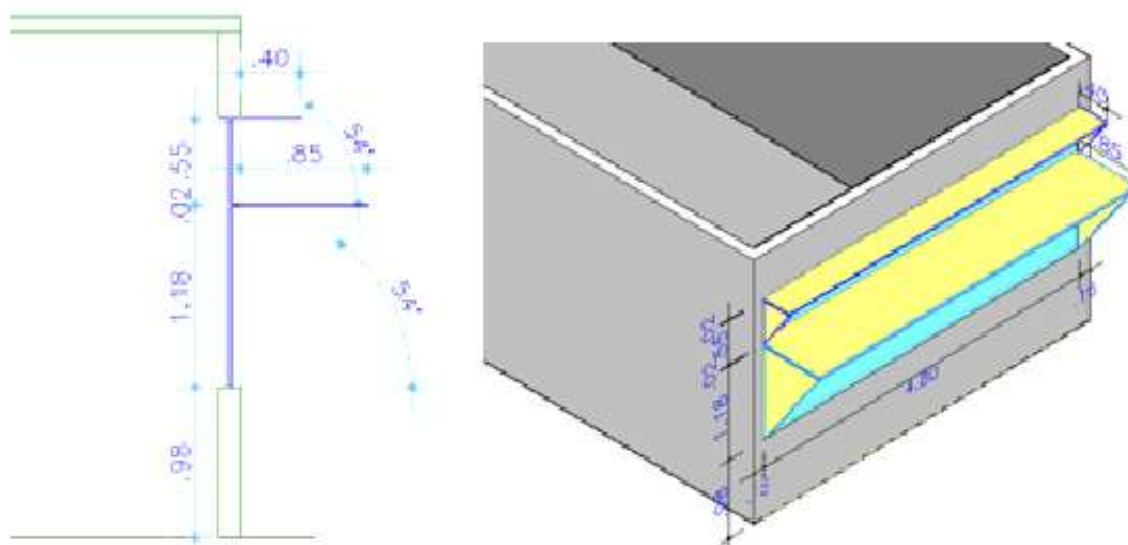
Figura 54 - Corte com detalhe da prateleira e dos ângulos de proteção gerados e para a volumetria do ambiente com a prateleira de luz
