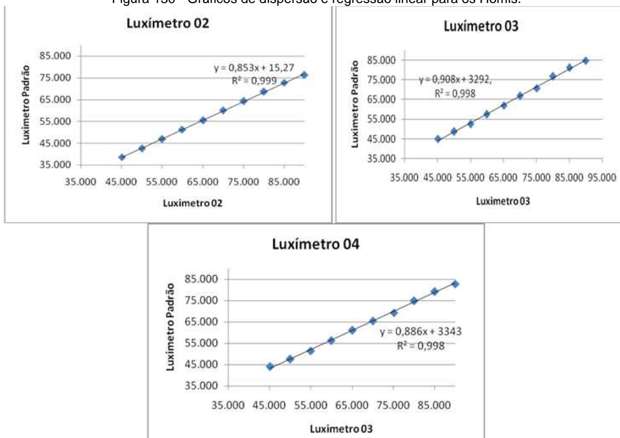
Figura 130 - Gráficos de dispersão e regressão linear para os Homis.
