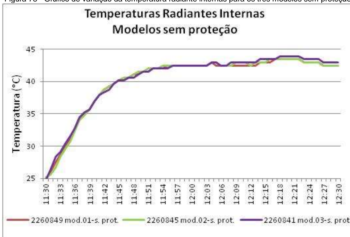
Figura 78 - Gráfico de variação da temperatura radiante internas para os três modelos sem proteção
