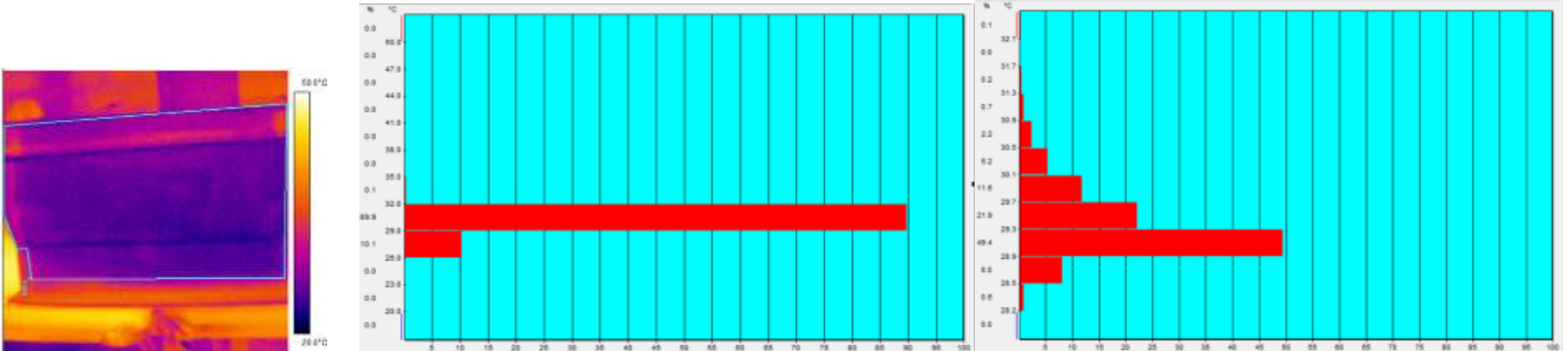
Figura 93 - Imagem térmica e histograma para temperaturas superficiais no início do aquecimento com brise
