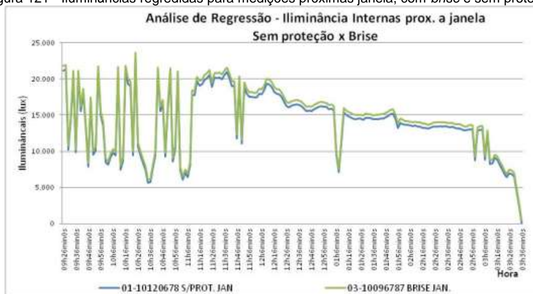
Figura 121 - Iluminâncias regredidas para medições próximas janela, com brise e sem proteção.
