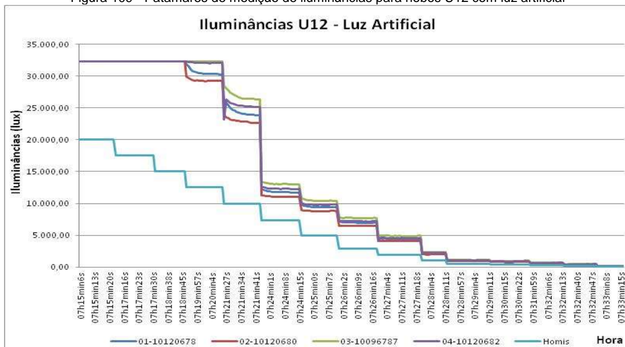
Figura 109 - Patamares de medição de iluminâncias para hobos U12 com luz artificial
