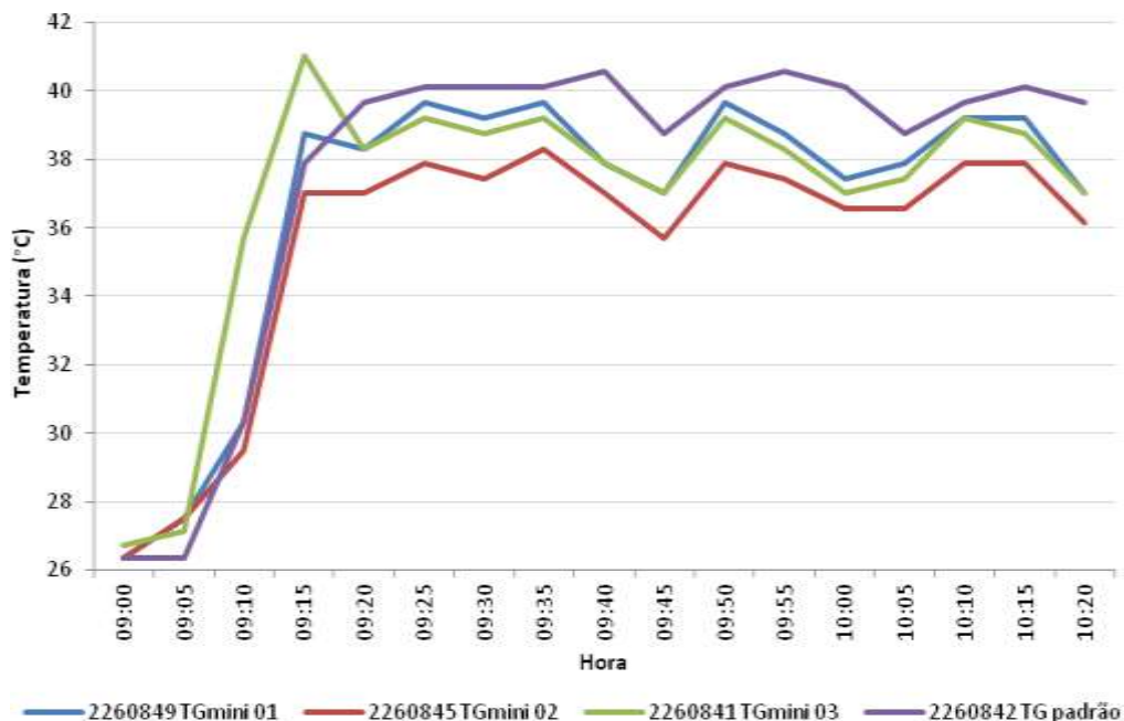
Figura 70 - Variação das temperaturas radiantes para regressão – dados brutos
