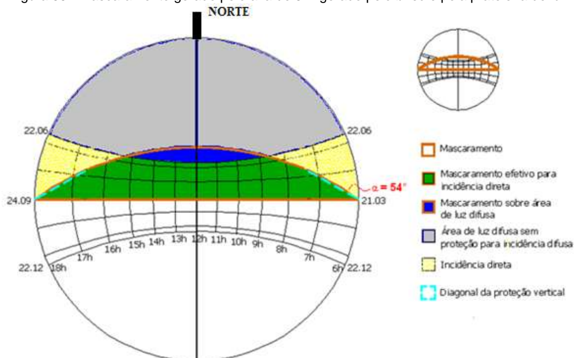
Figura 55 - Mascaramento gerado pelo alfa de 54° gerado pelo brise e pela prateleira de luz
