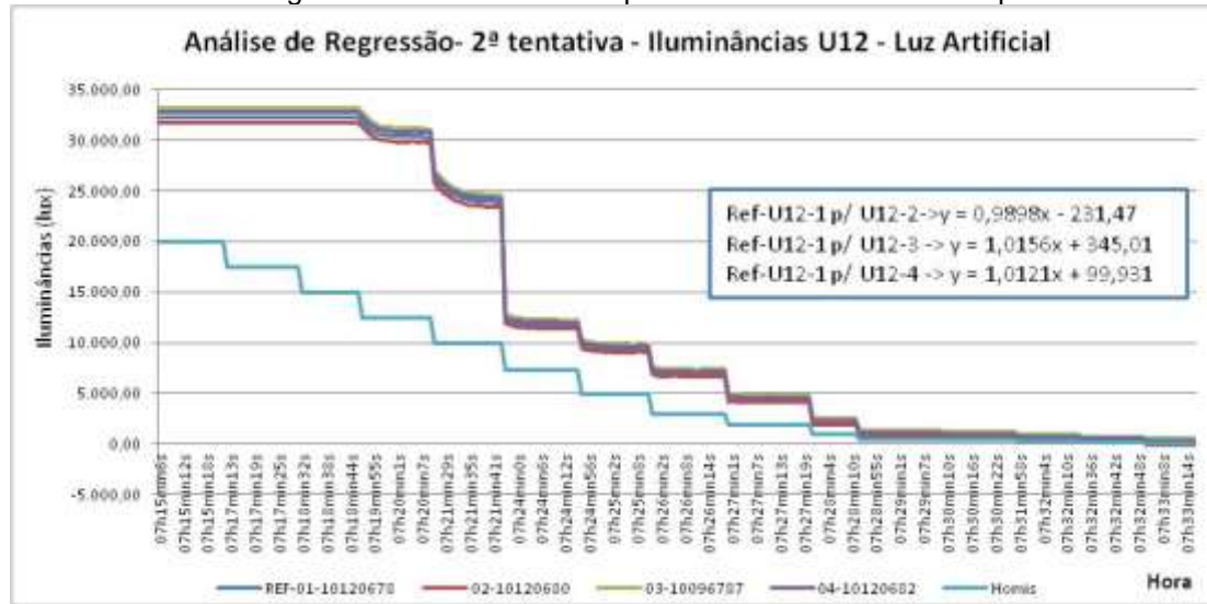
Figura 111 - Gráfico de Regressão das Iluminâncias para sensores U12 com a expressão da 2ª tentativa
