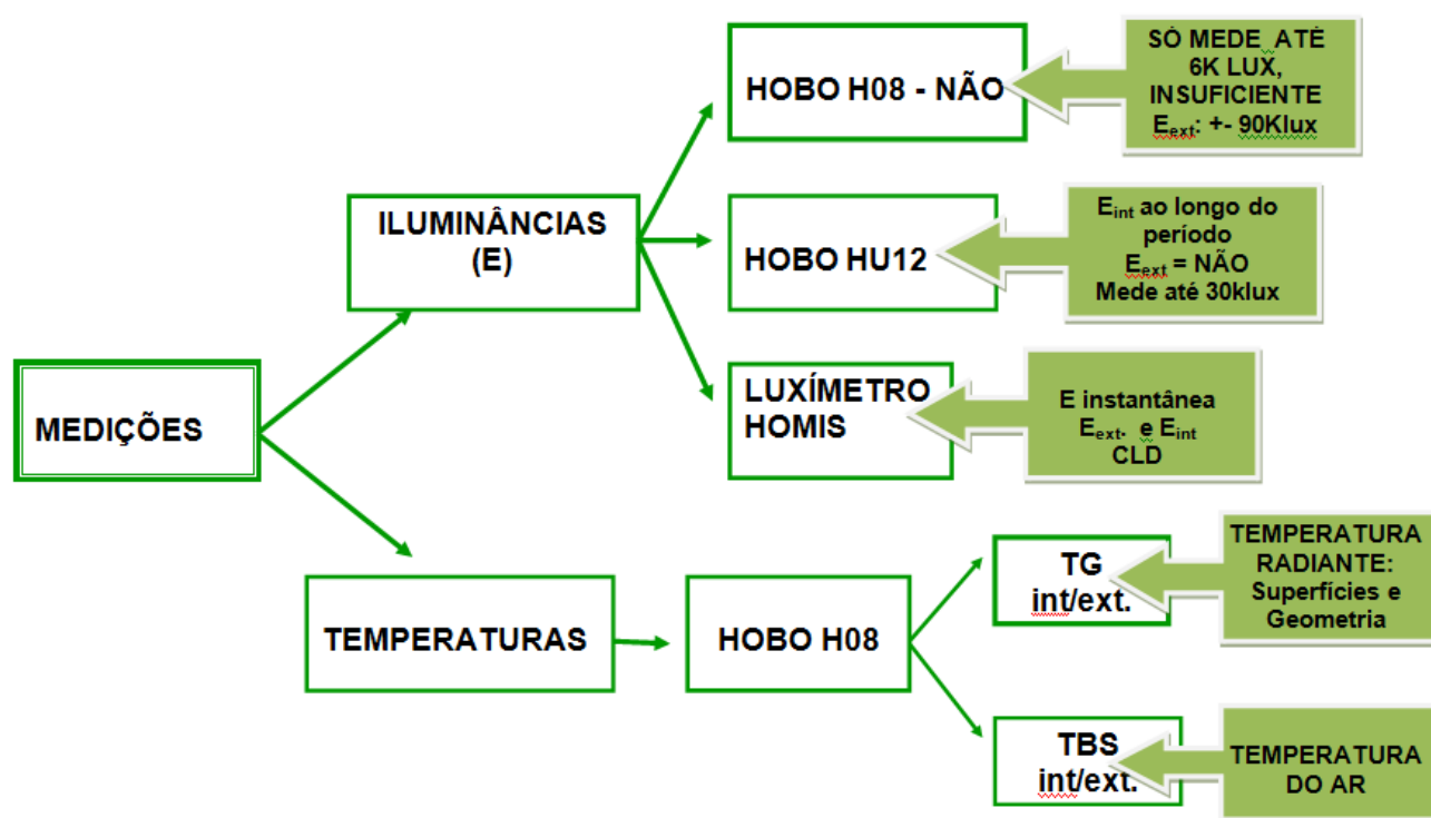
Figura 33 – Diagrama de tipos de sensores.
