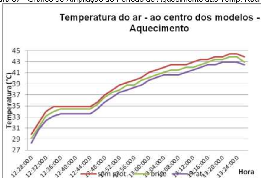
Figura 87 - Gráfico de Ampliação do Período de Aquecimento das Temp. Radiantes
