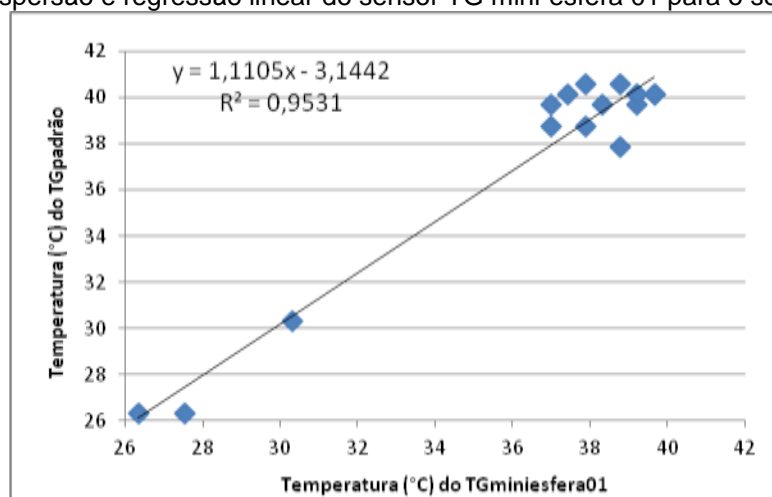
Figura 71 - Dispersão e regressão linear do sensor TG mini-esfera 01 para o sensor TGpadrão
