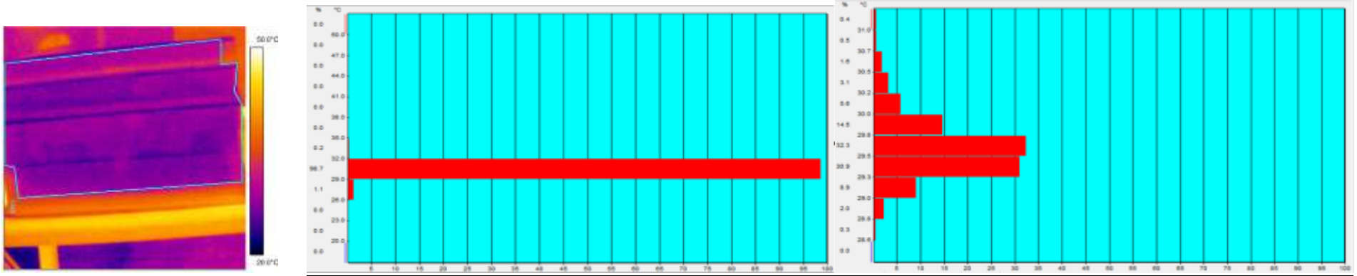
Figura 95 - Imagem térmica e histograma para temperaturas superficiais no início do aquecimento com prateleira
