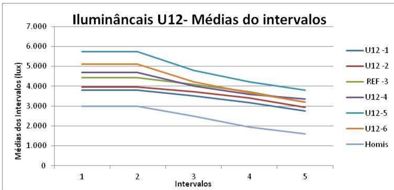
Figura 105 - Gráfico das Médias das iluminâncias dos intervalos
