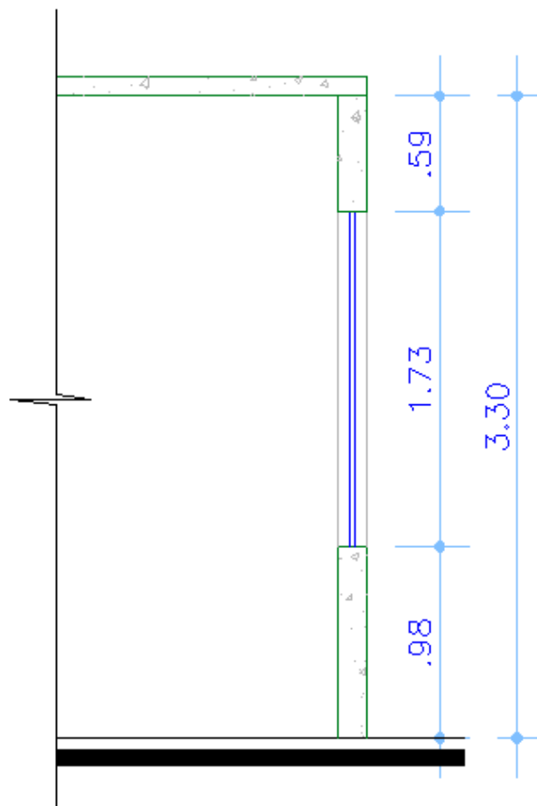
Figura 51 - Corte da janela
