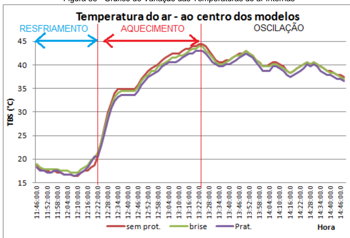
Figura 86 - Gráfico de Variação das Temperaturas do ar Internas
