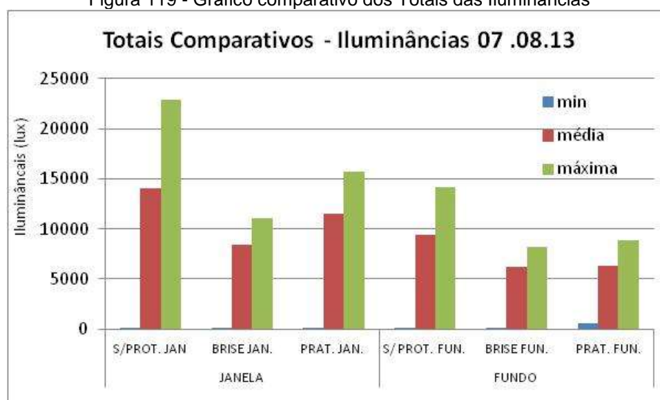
Figura 119 - Gráfico comparativo dos Totais das Iluminâncias
