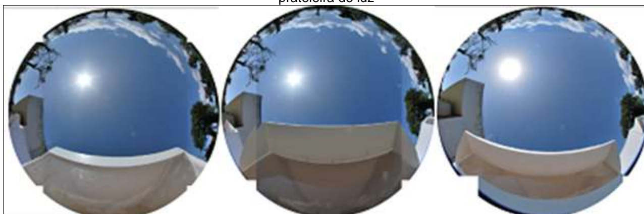
Figura 31 - Foto lente olho-de-peixe, à esquerda sem proteção, ao centro com brise e à direita com prateleira de luz
