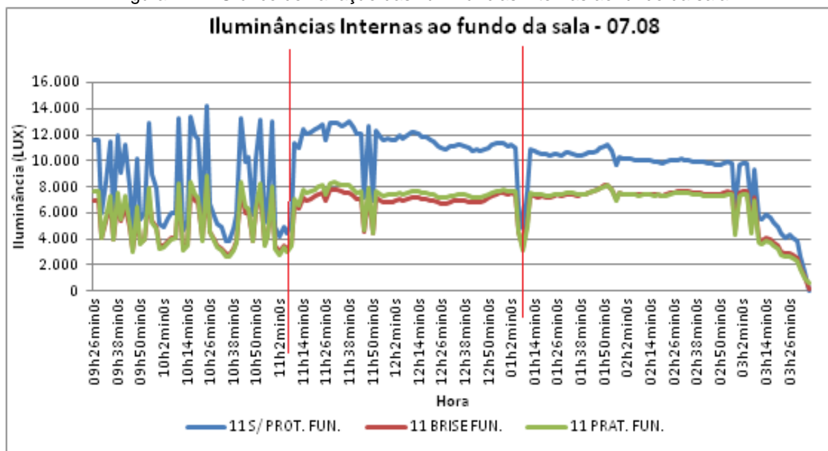
Figura 117 - Gráfico de variação das iluminâncias internas ao fundo da sala
