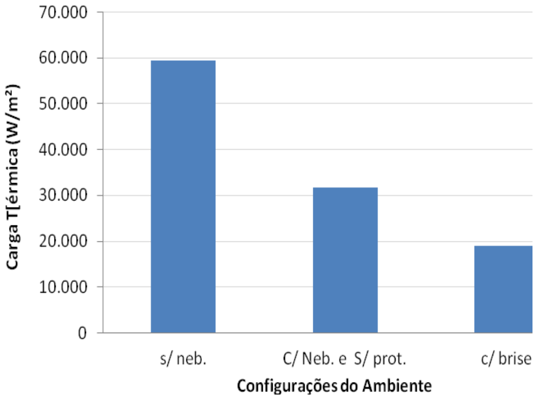
Figura 57 - Totais de ganhos de calor solar para a fachada norte, dia 22 de junho, Nebulosidade 6.1 – dados do programa Arqutrop e luz do sol.
