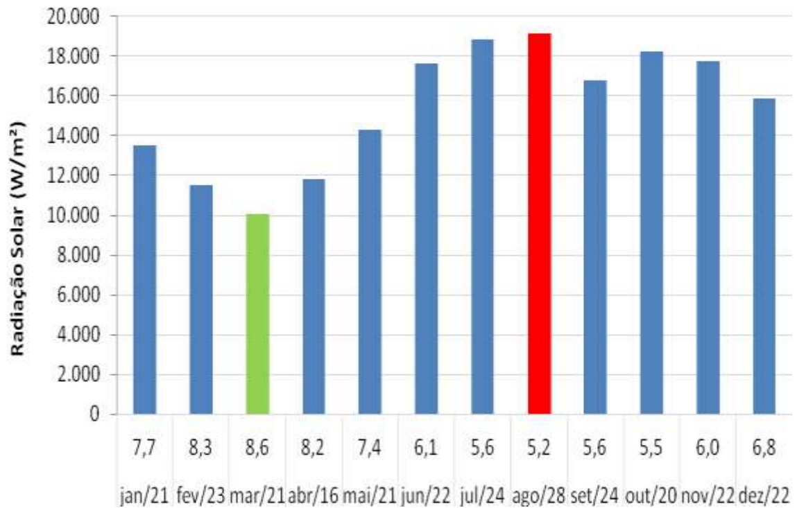
Figura 44 - Variação Anual da Carga Térmica Incidente Diária para Belém
