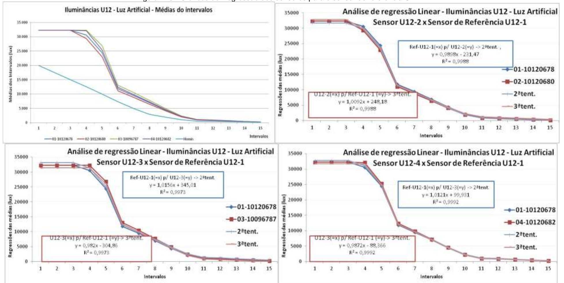
Figura 110 - Gráficos de Regressão dos sensores para o sensor de referência U12-1
