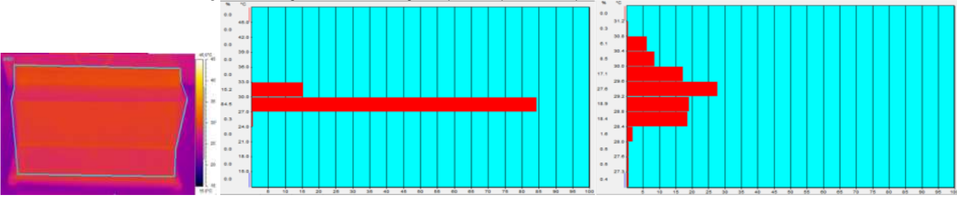
Figura 94 - Imagem térmica e histograma para temperaturas superficiais com brise, já aquecido.
