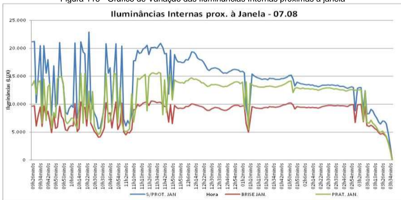
Figura 116 - Gráfico de Variação das Iluminâncias Internas próximas a janela
