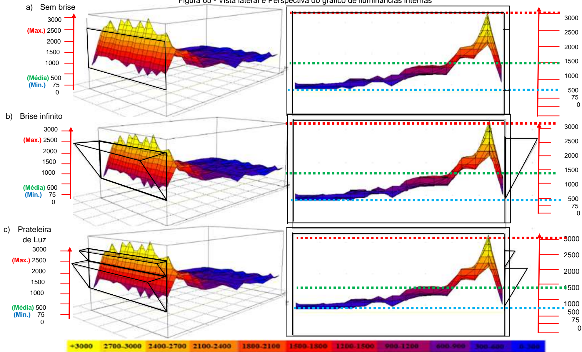
Figura 65 - Vista lateral e Perspectiva do gráfico de iluminâncias internas
