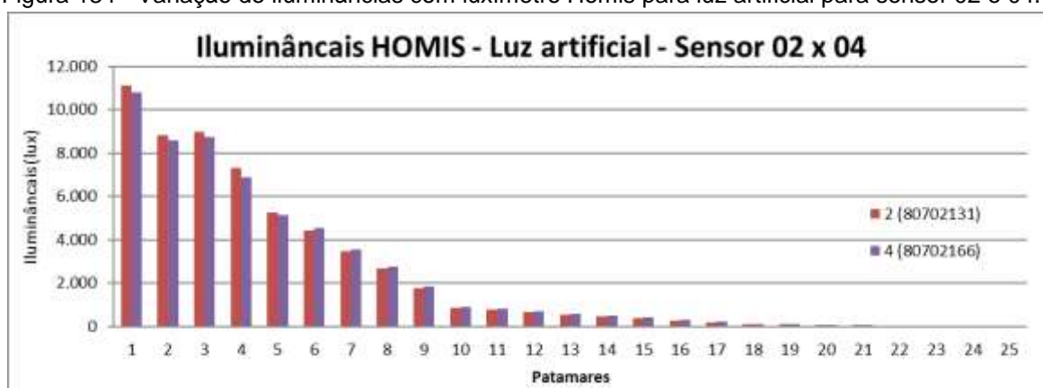
Figura 134 - Variação de iluminâncias com luxímetro Homis para luz artificial para sensor 02 e 04.
