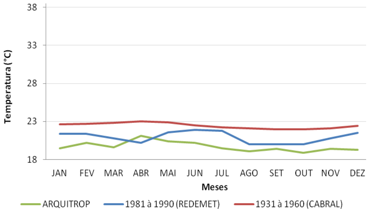
Figura 38 - Variação anual das temperaturas mínimas
