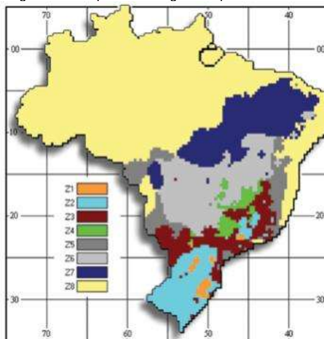
Figura 35 - Mapa climatológico simplificado do Brasil
