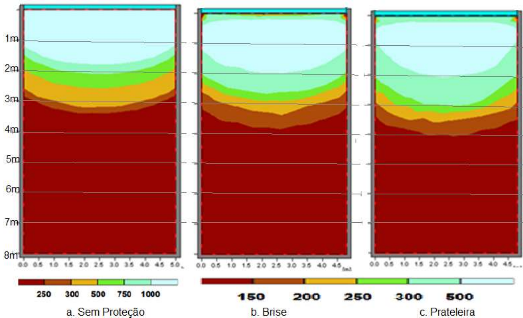
Figura 67 - Níveis de Iluminância em planta (pseudo cores) para luz direta, a esquerda: recinto sem proteção, ao centro com brise e à direita: com prateleira de luz
