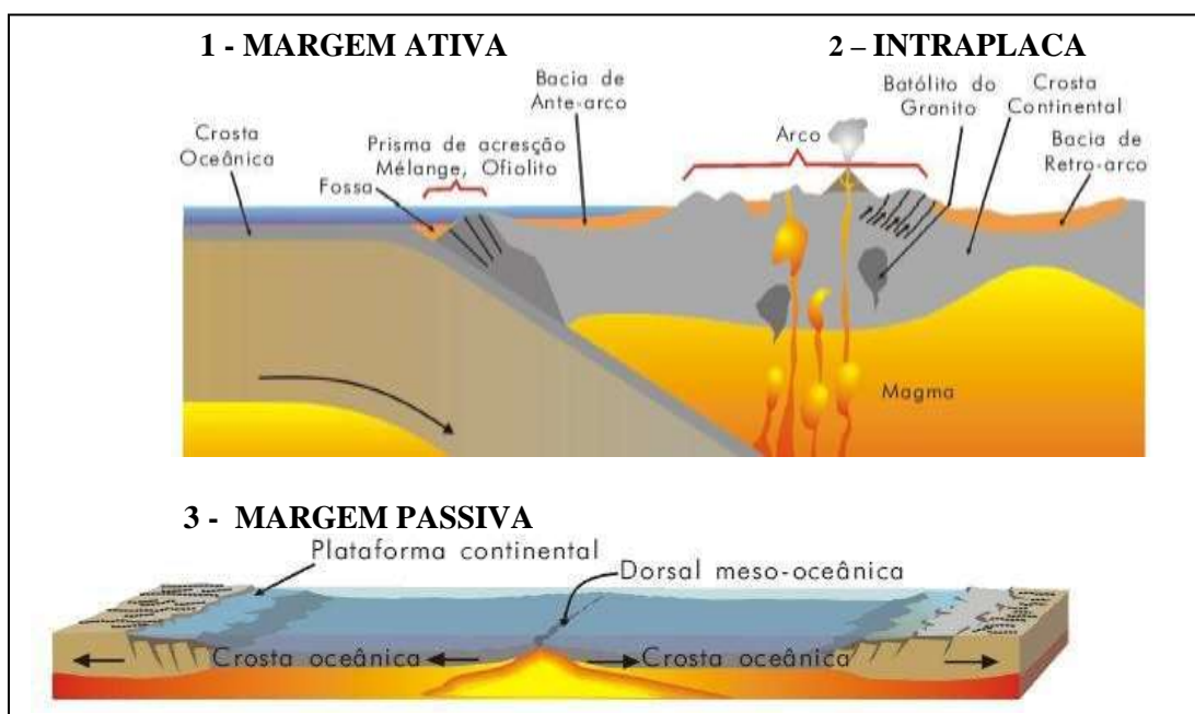
Figura 4.2 Principais tipos de relações entre as placas tectônicas. 1) Subducção de crosta oceânica; 2) Formação de um Arco-de-Ilhas e 3) Expansão de fundos oceânicos em dorsal meso-oceânica e fragmentação de uma massa continental pelo desenvolvimento de margens passivas.
