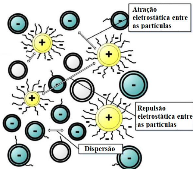
Figura 2.5. Representação esquemática do mecanismo de dispersão dos superplastificantes com base de policarboxilato Fonte: Carvalho (2015) - adaptado.
