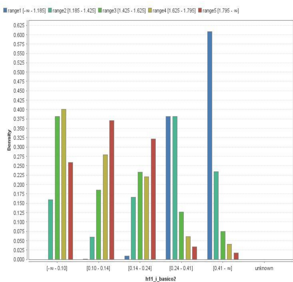
Figura 32 - Densidade de probabilidade dos intervalos discretizados do THDv em relação a corrente do 11º harmônico.
