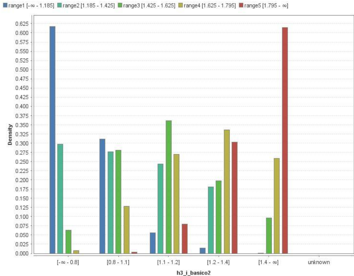
Figura 30 - Densidade de probabilidade dos intervalos discretizados do THDv em relação a corrente do 3º harmônico.
