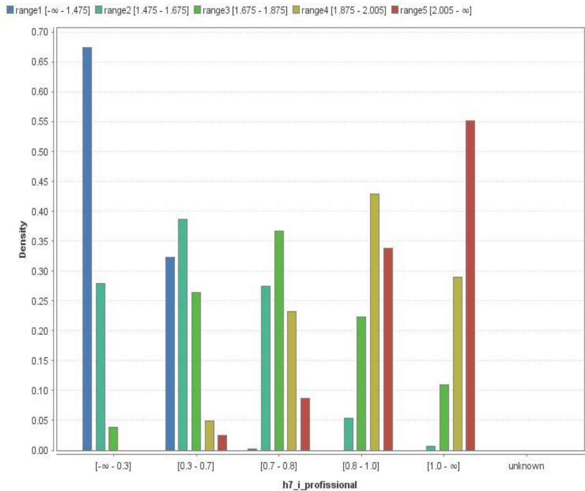
Figura 40 - Densidade de probabilidade dos intervalos discretizados do THDv em relação a corrente do 7º harmônico.
