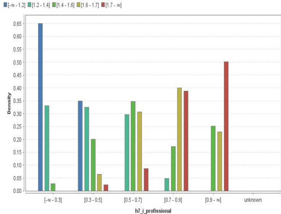
Figura 24 - Densidade de probabilidade dos intervalos discretizados do THDv em relação a corrente do 7º harmônico.
