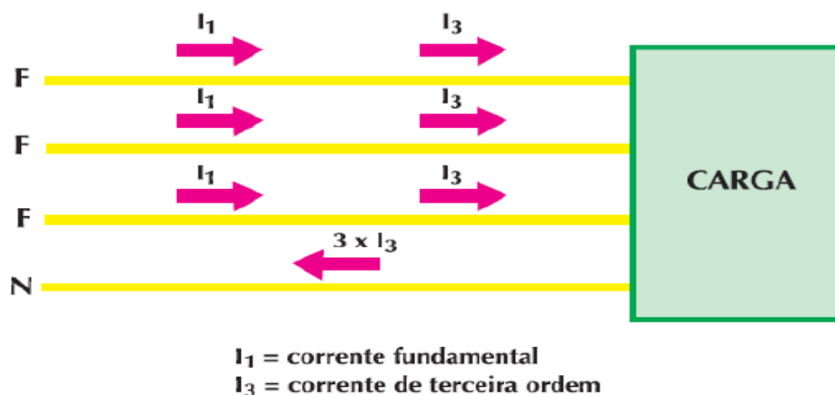
Figura 2 - Harmônico de sequência zero.
