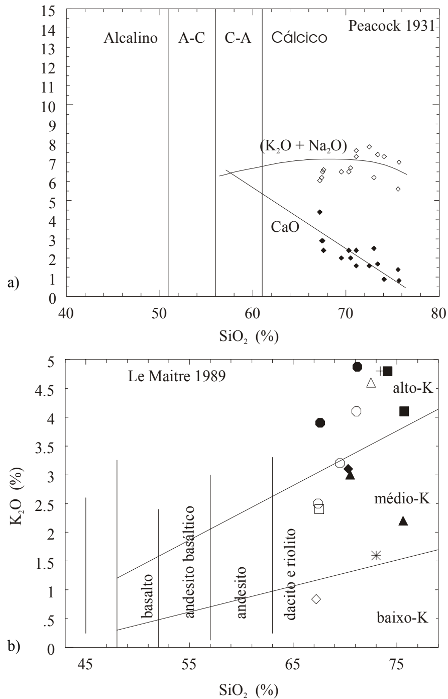
Figura 5.4. a) Diagrama SiO 2 vs. CaO e Na 2 O + K 2 O (cf. Peacock 1931), A-C (Álcali-Cálculo), C-A (Cálculo-Alcalino). b) Diagrama SiO 2 vs. K 2 O (cf. Le Maitre 1989). Símbolos como na figura 5.1.
