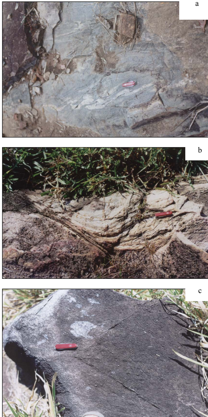
Figura 3.8. a) Hb Mzg (JP-10) com dobras ptigmáticas desenhadas por veios quartzo-feldspáticos. b) Hb Mzg (JP-10) com dobras abertas. c) Hb Tonal (JP-41) com pares conjugados de deformação.
