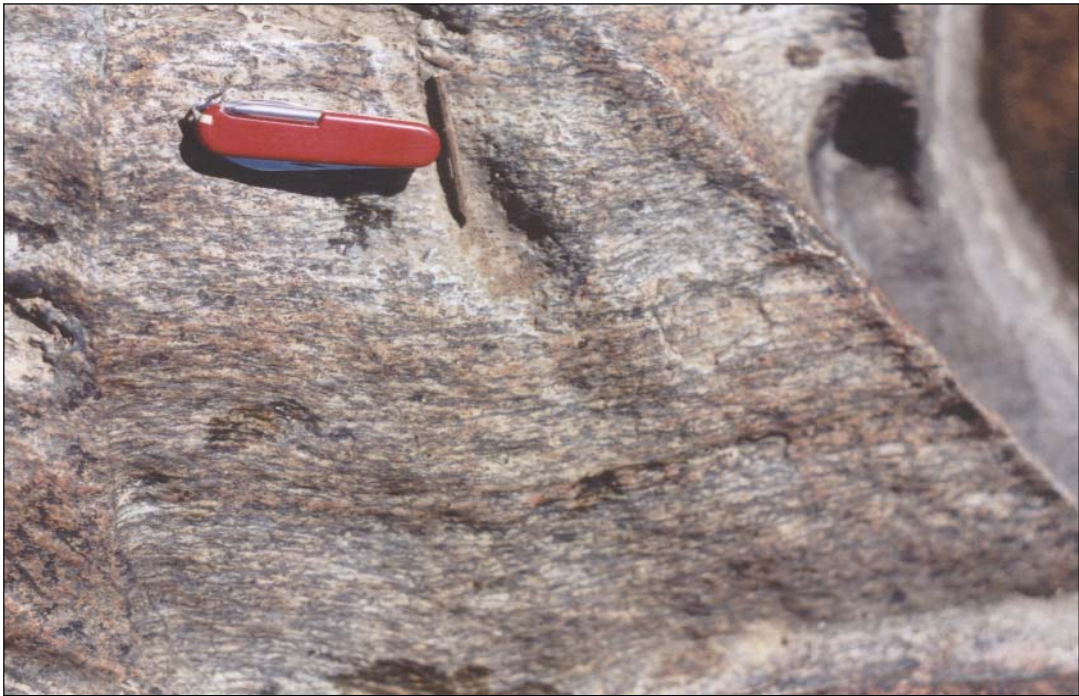
Figura 3.4. Detalhe da foliação fortemente penetrativa desenvolvida em Biotita Granodiorito (JP-23).
