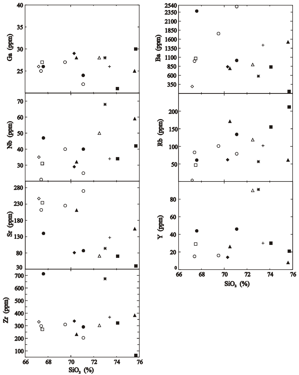
Figura 5.2. Diagramas de variação sílica vs. elementos-traço para as rochas estudadas. Símbolos como na figura 5.1.
