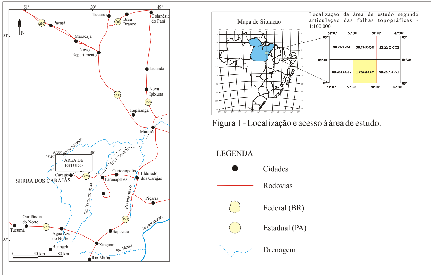
Figura 1. Mapa de localização da área de estudo (em destaque).
