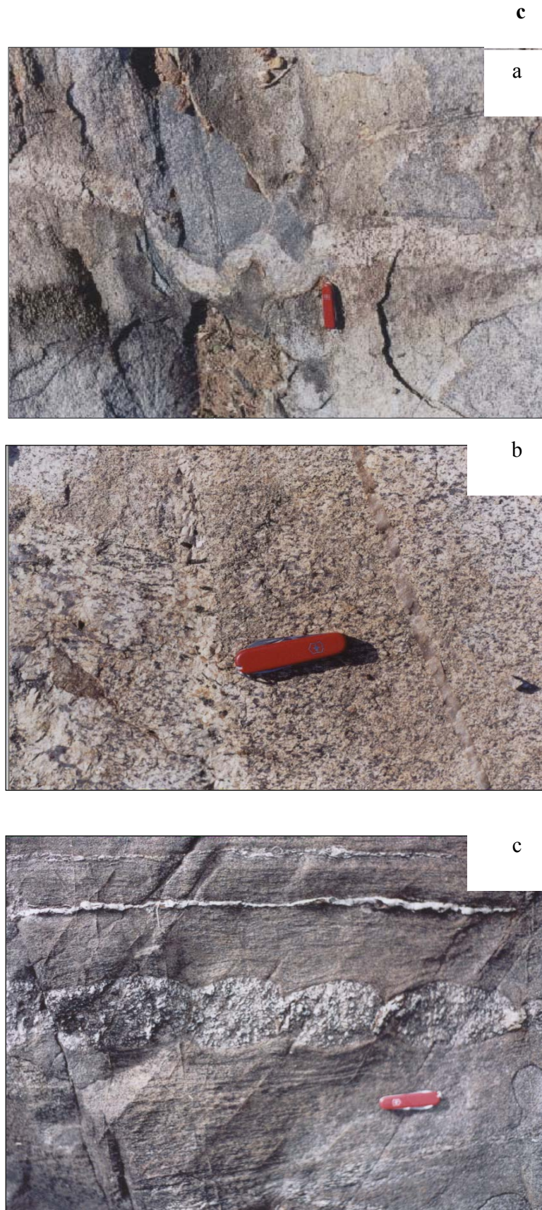
Figura 3.7. Veios quartzo-feldspáticos cortando granito: a) veio levemente dobrado (Bt Mzg, JP-29); b) veio com cristais de anfibólio orientados segundo a foliação (Hb Mzg, JP-30). c) feições do tipo pinch-and-swell (Hb Mzg, JP-10).
