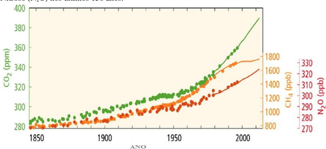
Figura 3 – Aumento das concentrações do Dióxido de Carbono (CO 2 ), Metano (CH 4 ) e Óxido Nitroso (N 2 O) nos últimos 150 anos.
