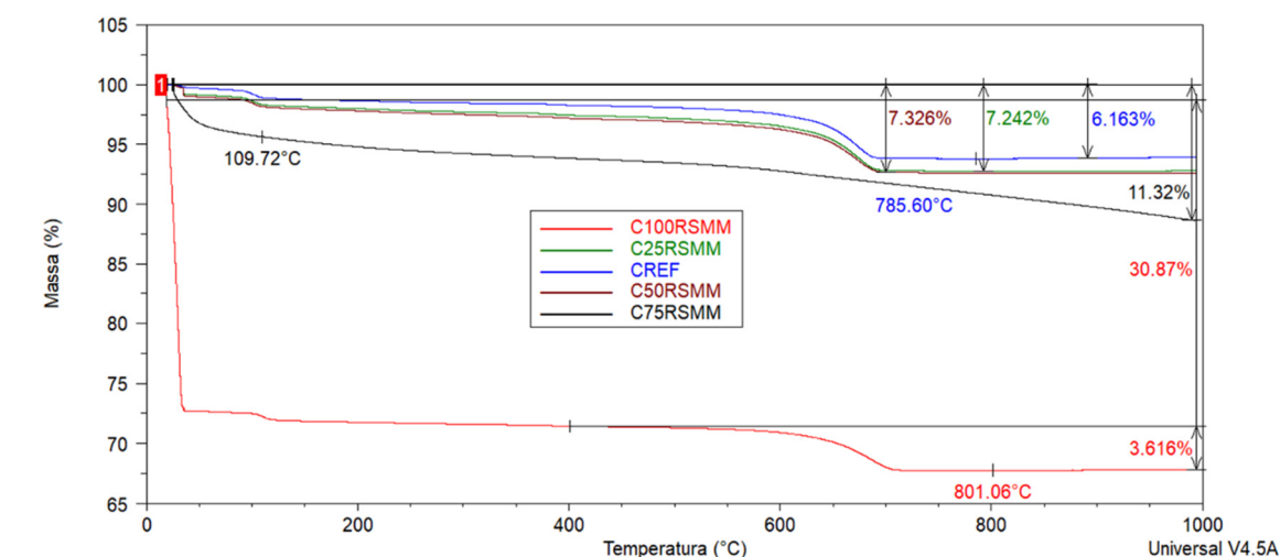
Figura 30 – Análise termogravimétrica das argamassas
