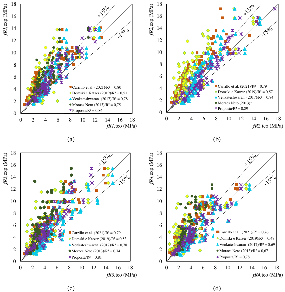
Figura 7.2. Gráfico de dispersão de resultado experimental-teórico, f_{Ri,exp}/f_{Ri,teo} : (a) f_{R1,exp}/f_{R1,teo} ; (b) f_{R2,exp}/f_{R2,teo} ; (c) f_{R3,exp}/f_{R3,teo} ; (d) f_{R4,exp}/f_{R4,teo} .
