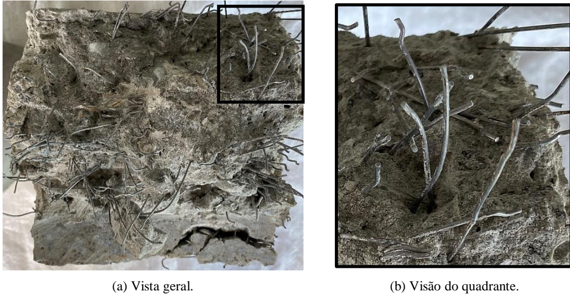
Figura 6.1. Seção transversal A_p do prisma com volume de fibra igual à 1,5%.
