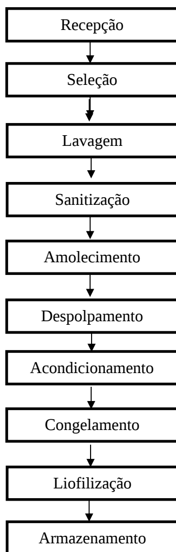
Figura 2. Fluxograma da descrição do processo de despulpamento de açaí dos acessos de Euterpe oleracea e Euterpe precatoria . Fonte: Autor, 2022.
