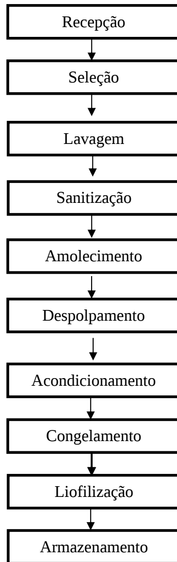
Figura 1. Fluxograma do processo de despulpamento de açaí dos acessos de Euterpe oleracea e Euterpe precatoria . Fonte: Autor (2022).
