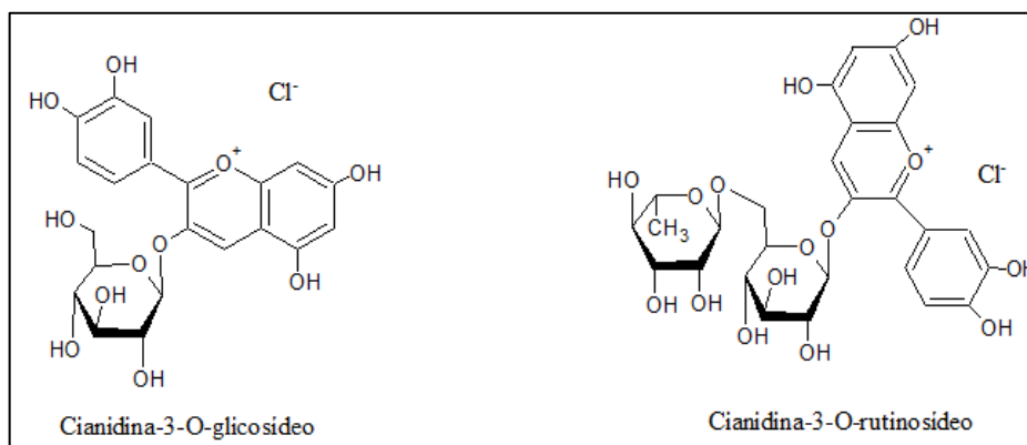
Figura 4. Estrutura química das principais antocianinas encontradas no açai. Fonte: Autor (2022).
