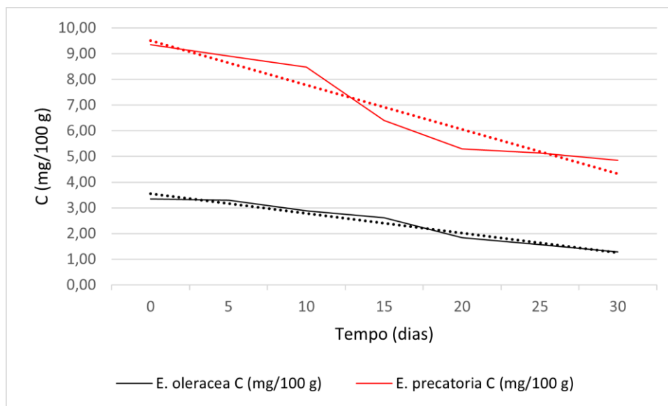
Figura 8. Modelo de primeira ordem ajustado pelo curva de degradação analisando os resultados da concentração de antocianinas monoméricas totais em função do tempo para as balas de goma com açaí liofilizado de Euterpe oleracea e de Euterpe precatoria (Model: V2=C0*Exp(-k*V1) ).
