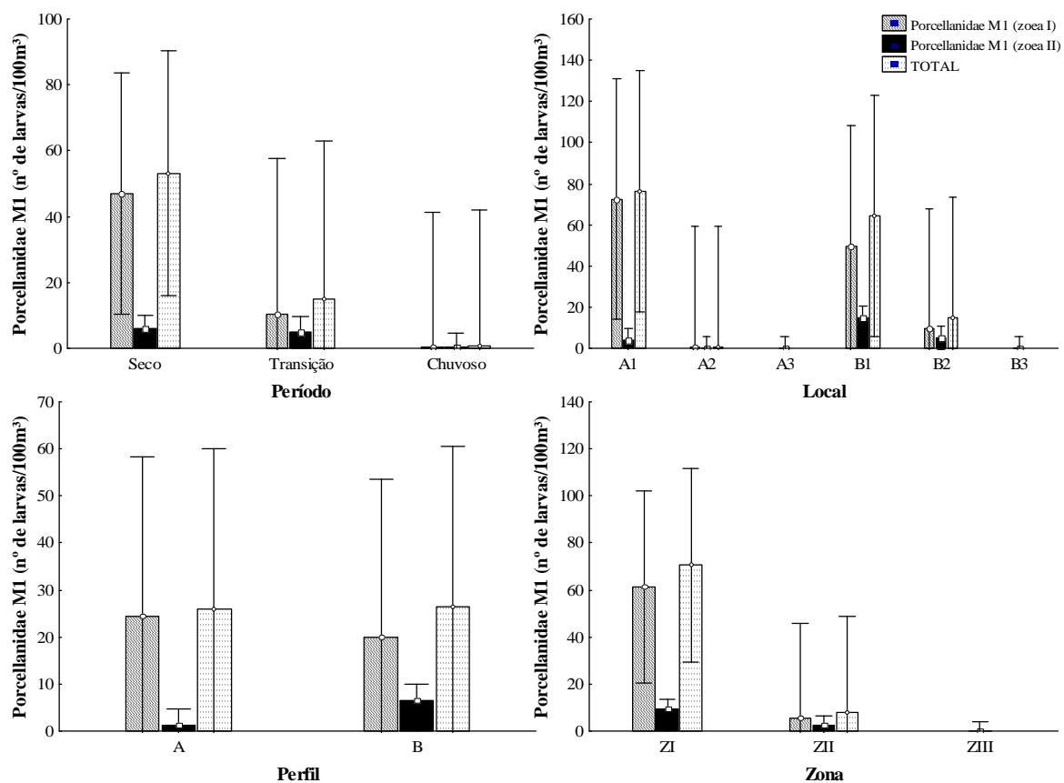
FIGURA 10: Densidade larval média (n° de larvas/100m³) do morfotipo de Porcellanidae nos estágios de zoea I, zoea II e em ambos os estágios (total); em relação aos períodos, locais, perfis e zonas do estuário do Rio Marapanim, PA. Barras verticais: média \pm intervalo de confiança (95%). M1= morfotipo 1.
