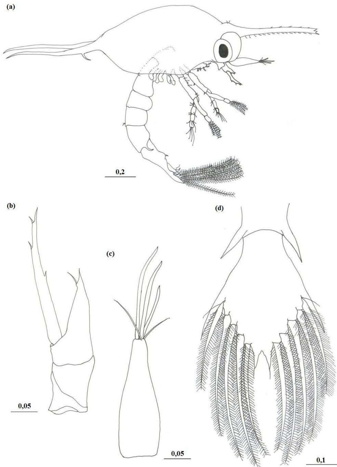
FIGURA 1: Apêndices larvais de Porcellanidae Morfotipo 1 ( zoea I). (a) Porcellanidae Morfotipo 1 ( zoea I); (b) antena; (c) antênula; (d) télson. Escala em milímetros (mm). Rostro representado truncado.
