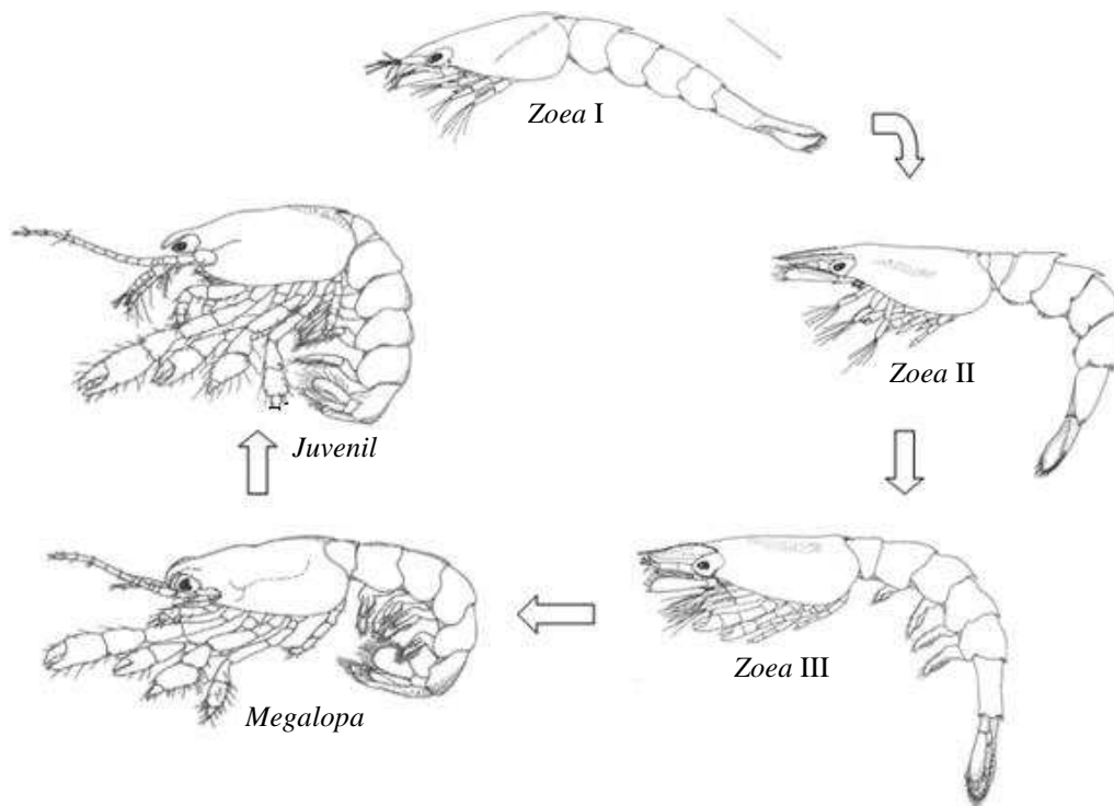
FIGURA 3: Representação dos estágios larvais de Lepidophthalmus siriboia (Axiidea). Modificado de Abrunhosa et al. (2005).
