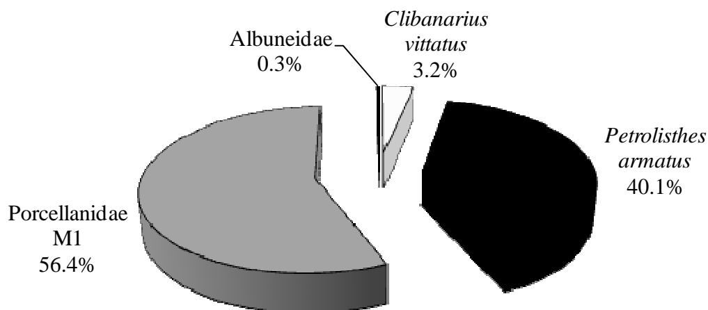
FIGURA 5: Contribuição percentual das larvas de Anomura coletadas no estuário do Rio Marapanim (PA) no período de agosto de 2006 a julho de 2007. M1 = morfotipo de Porcellanidae.
