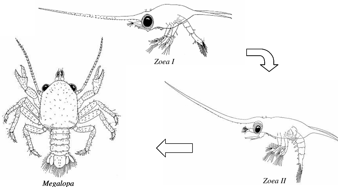
FIGURA 2: Representação dos estágios de desenvolvimento larval de Petrolisthes tridentatus (Porcellanidae). Modificado de Gore (1971a).
