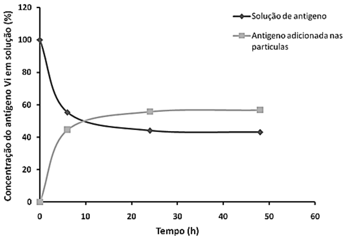
Figura 18: Gráfico da cinética de adsorção do antígeno Vi em solução nas nanopartículas de quitosana 1,0% - 1,0% (QS - PMAA).
