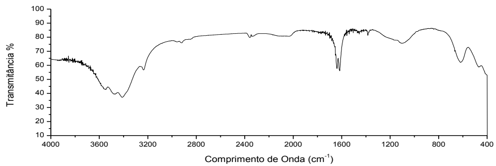
Figura 10: Espectro de Infravermelho do amostra 2 (cepas mortas por acetona).
