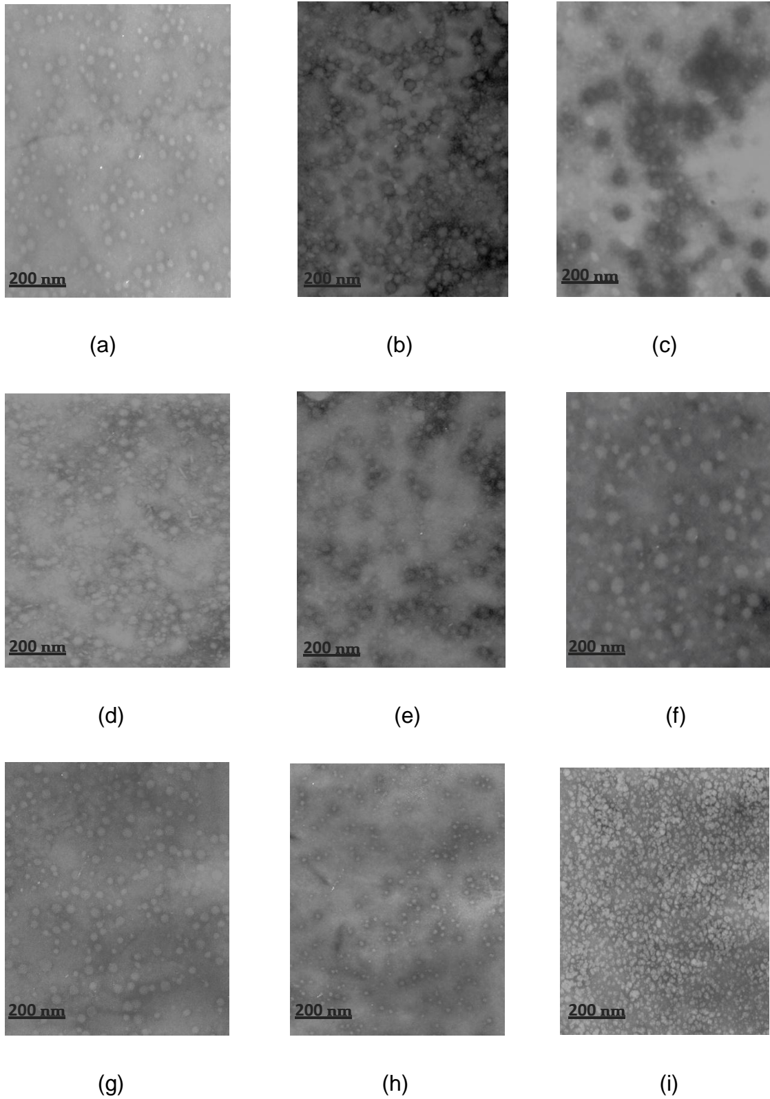
Figura 15: Microscopia eletrônica de transmissão das nanopartículas de quitosana. a) 0,5% - 0,5% (QS - PMAA); b) 0,8% - 0,5%; c) 1,0% - 0,5%; d) 0,5% - 0,8%; e) 0,8% - 0,8%; f) 1,0% - 0,8%; g) 0,5% - 1,0%; h) 0,8% - 1,0%; i) 1,0% - 1,0%.
