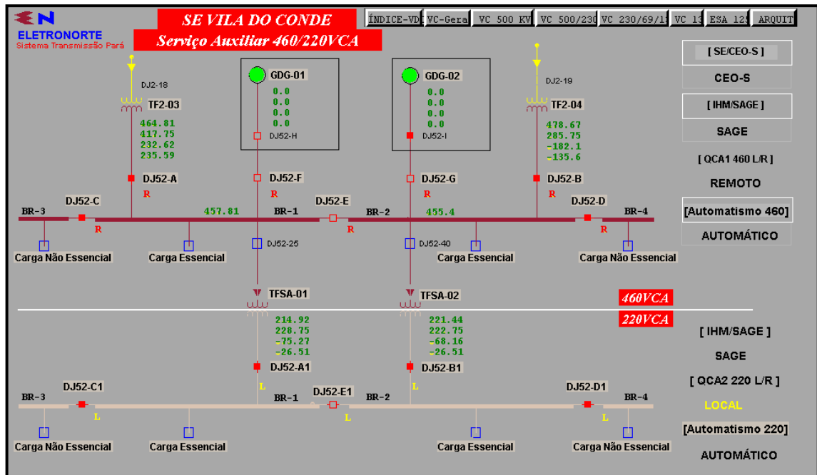
Fig.08. Diagrama Unifilar ESA 460/220 VCA da SE VDC
