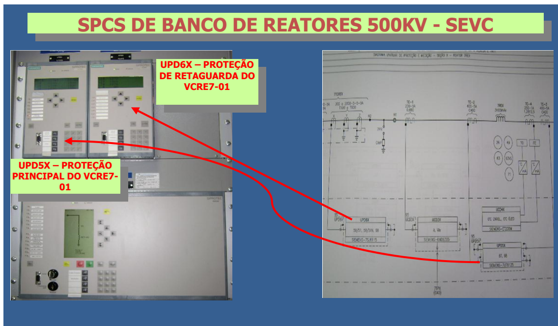
Fig.10. SPCS de Banco de Reatores da SE VDC
