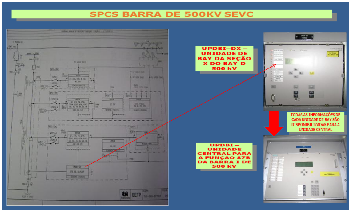
Fig.11. SPCS Barra de 500KV da SE VDC
