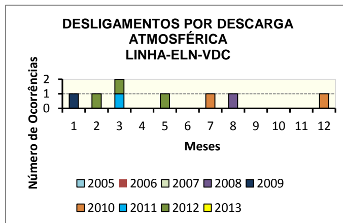
Gráfico. 02. Desligamentos na Linha de Transmissão Produzidos por Descarga Atmosférica. Fonte: Sistema Eletronorte-Eletrobrás
