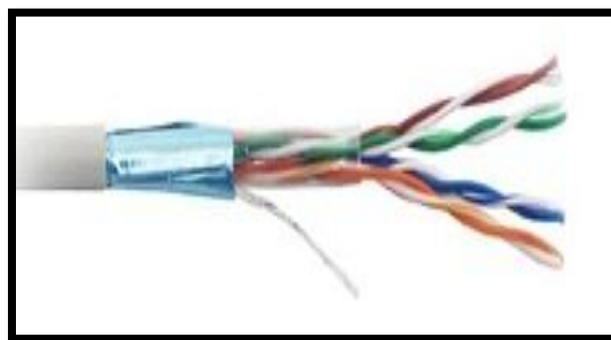
Fig.25. Cabo FTP. Fonte: Adaptada de Guia do Hardware
