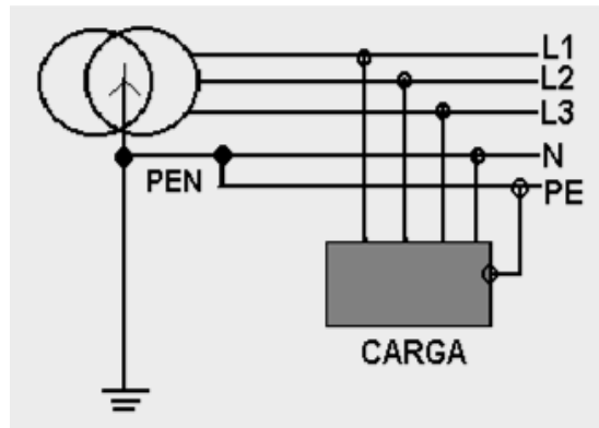
Fig.22. Esquema TN-C-S. Fonte: Adaptada de Procobre
