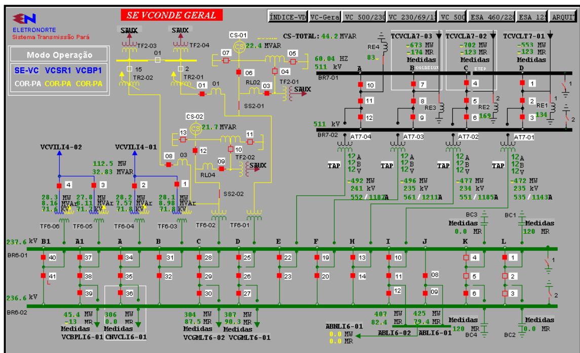
Fig.06. Diagrama Unifilar Elétrico da SE VDC
