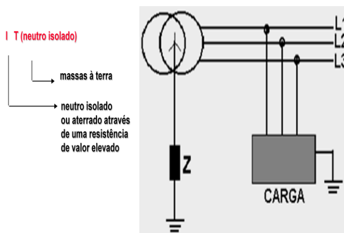
Fig.24. Esquema IT. Fonte: Adaptada de Procobre
