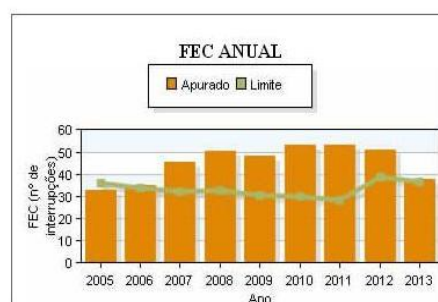
Gráfico. 05. FEC Anual. Fonte: ANEEL
