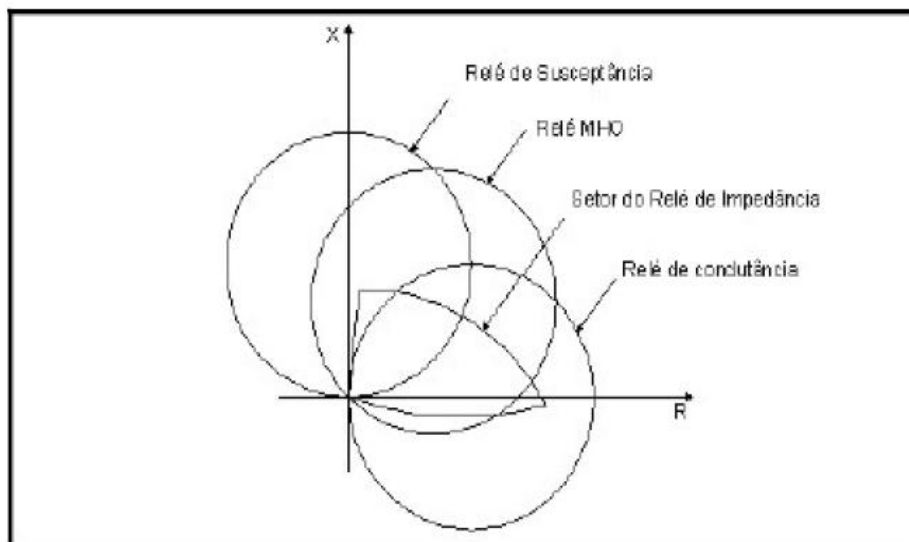
Fig.33. Características Gerais de Operação de Relés de Distância com Característica de Direcionalidade [18]
