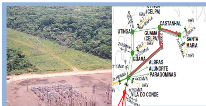
Fig.37. Subestação Vila do Conde com a Linha de Transmissão Vila do Conde – Castanhal, selecionada como piloto do sistema elétrico para aplicação da metodologia desenvolvida
