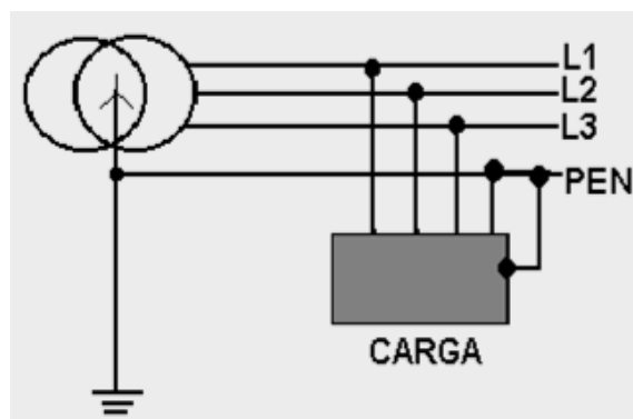
Fig.21. Esquema TN-C. Fonte: Adaptada de Procobre
