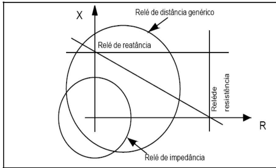
Fig.32. Características Gerais de Operação de Relés de Distância [18]
