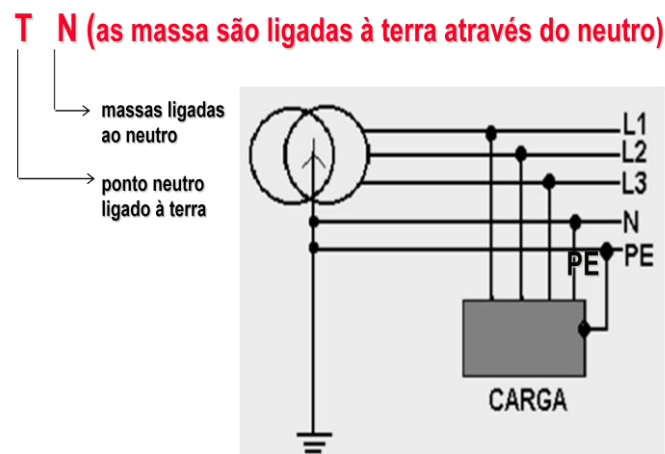
Fig.20. Esquema TN-S. Fonte: Adaptada de Procobre
