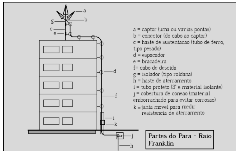
Fig.17. Sistema de Proteção por Para-raios Tipo Franklin. Fonte: Adaptada de Bohn.
