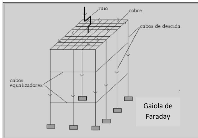
Fig.18. Sistema de Proteção Gaiola de Faraday. Fonte: Adaptada de Bohn.
