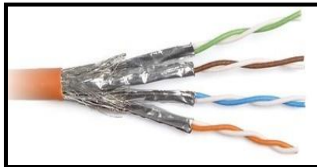
Fig.27. Cabo SSTP. Fonte: Adaptada de Guia do Hardware
