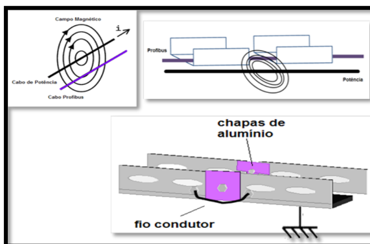
Fig.28. Bandeja Metálica Aterrada. Fonte: Adaptada de Artigo SMAR 2011
