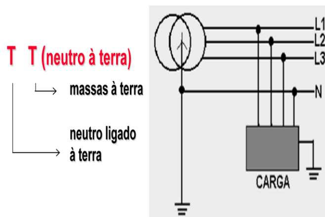
Fig.23. Esquema TT. Fonte: Adaptada de Procobre
