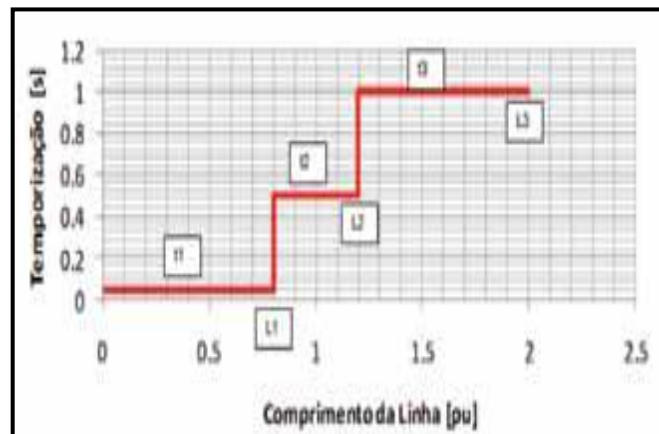
Fig.31. Temporizações das Zonas de Proteção. Fonte: Adaptada de http://www.osetoreletrico.com.br .
