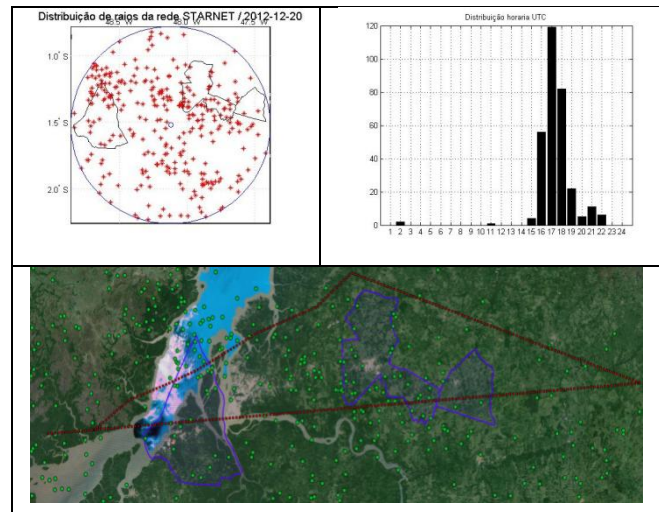
Fig.43. Dados de Raios em 20.12.12. Fonte: STARNET
