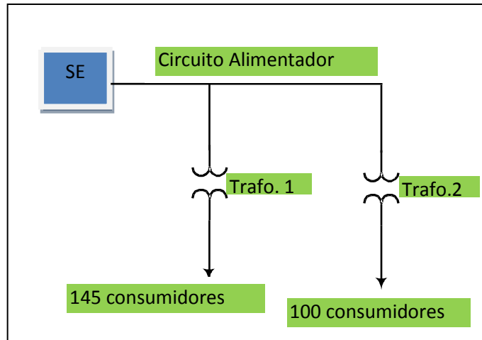
Fig.36. Circuito Alimentador
