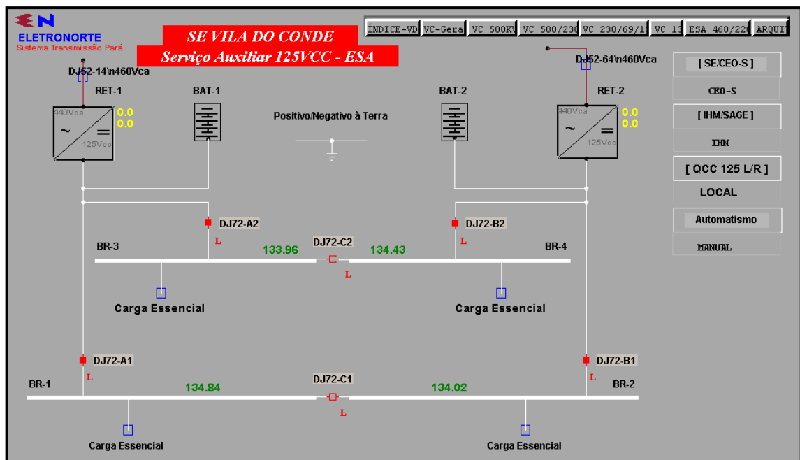
Fig.07. Diagrama Unifilar ESA 125 VCC da SE VDC
