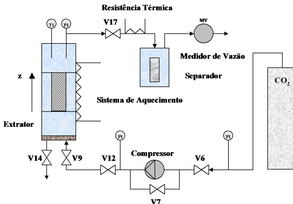
Figura 3.3 - Fluxograma simplificado da unidade de extração.
