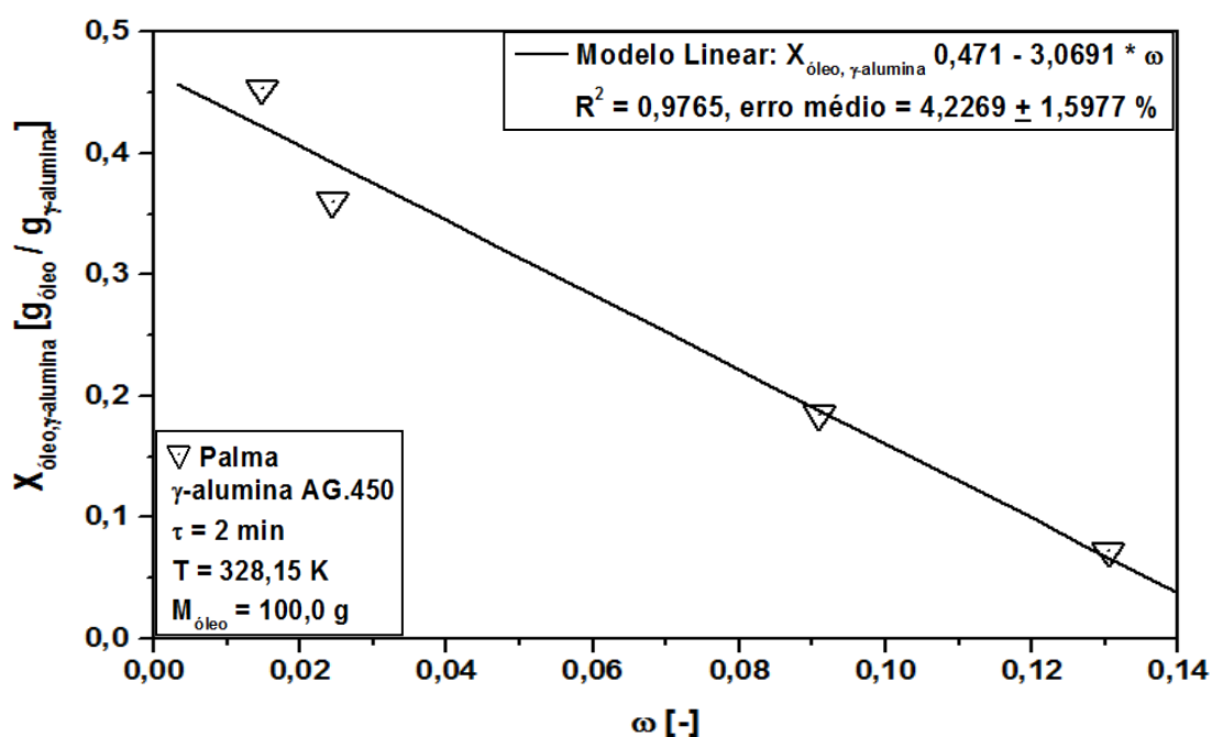
Gráfico 4.3 - Influência da fração mássica de \gamma -alumina AG.450 sobre a capacidade de adsorção do óleo de palma.
