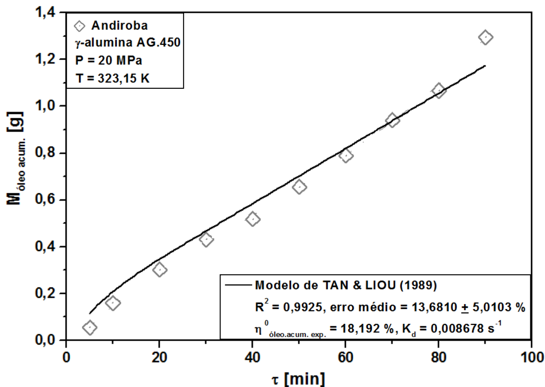
Gráfico 4.23 - Modelagem da curva de dessorção do óleo de andiroba \gamma -alumina AG.450 a 20 MPa e 323,15 K utilizando-se o modelo de Tan & Liou.
