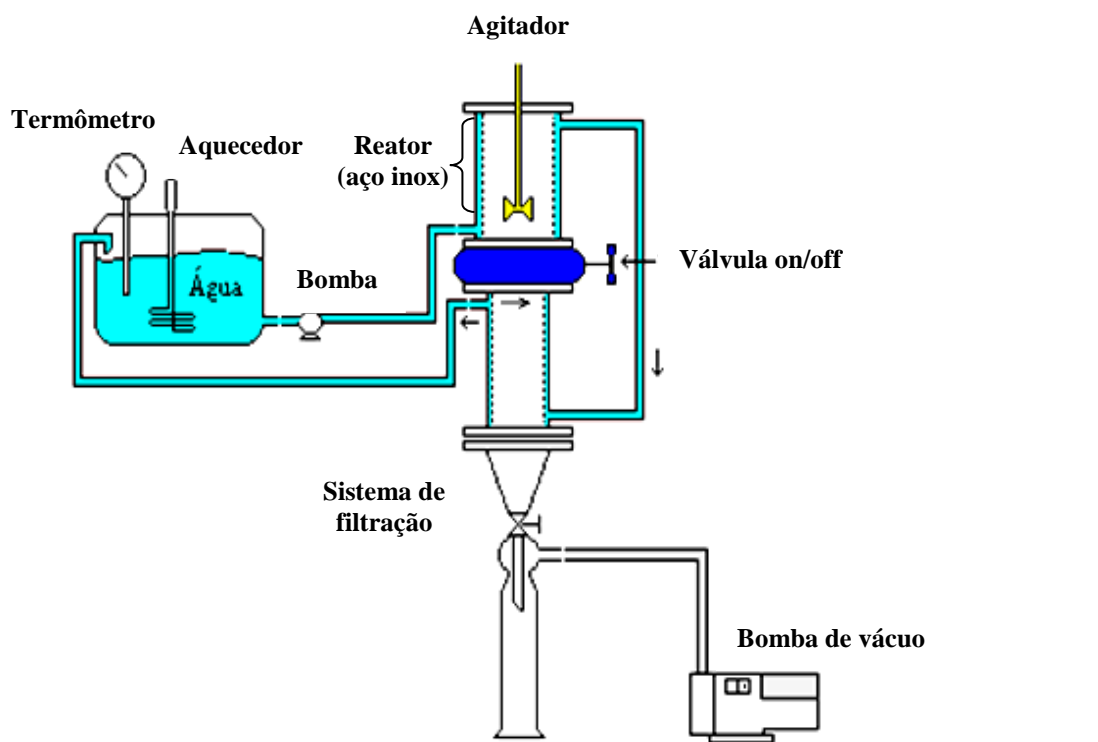
Figura 3.1 - Fluxograma simplificado da unidade de adsorção e filtração (RAIOL & ASSUNÇÃO, 1999).
