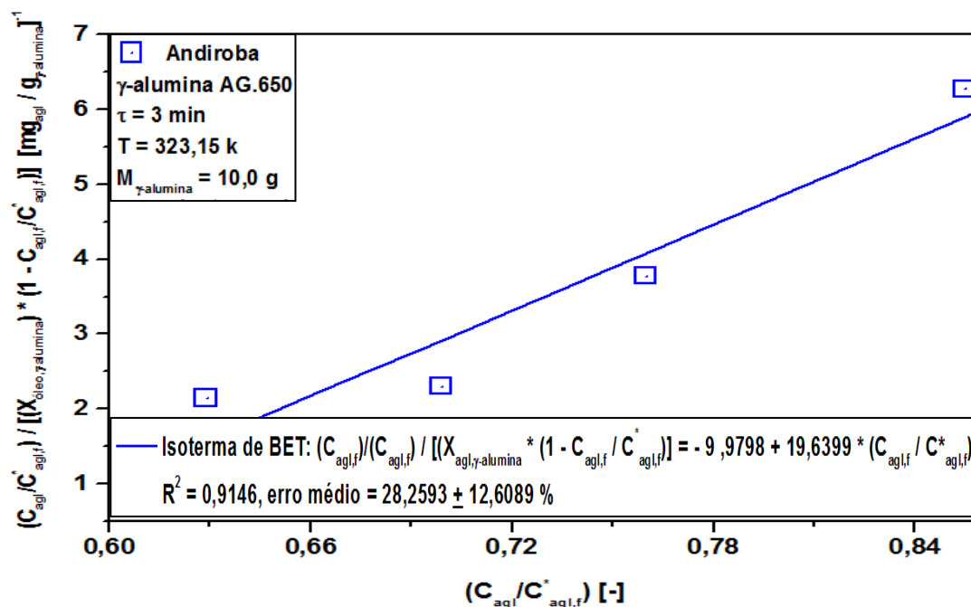
Gráfico 4.17 - Modelagem da isoterma do óleo de andiroba em \gamma -alumina AG.650 utilizando-se o modelo de BET.
