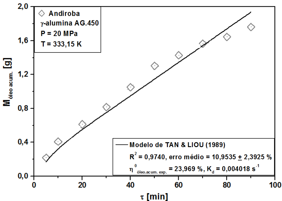
Gráfico 4.25 - Modelagem da curva de dessorção do óleo de andiroba \gamma -alumina AG.450 a 20 MPa e 333,15 K utilizando-se o modelo de Tan & Liou.
