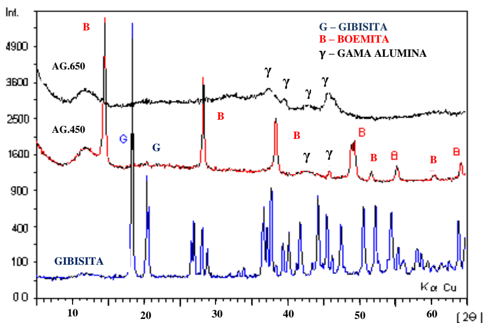
Gráfico 4.1 - Difração de raio-X após a ativação térmica do \text{Al}(\text{OH})_3 (AZEVEDO et al. 2011).
