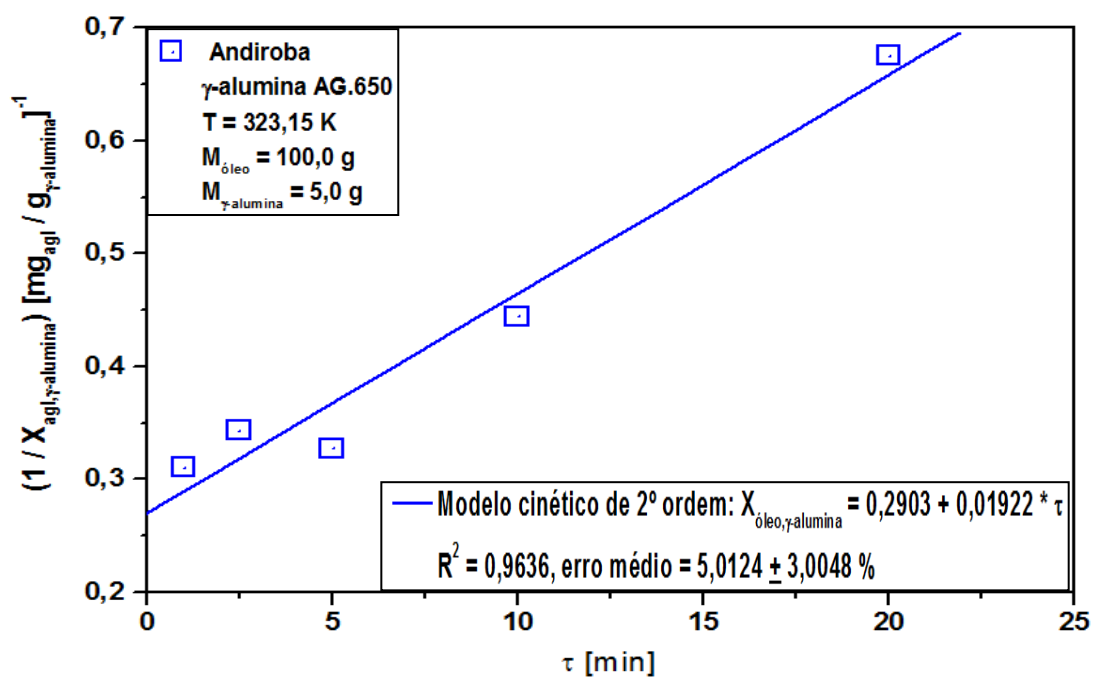
Gráfico 4.13 – Modelagem cinética de adsorção de ácidos graxos livres do óleo de andiroba em \gamma -alumina AG.650.
