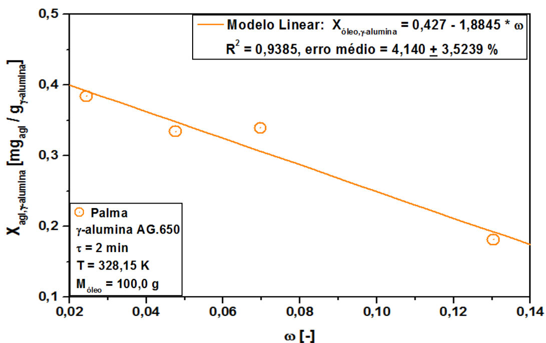
Gráfico 4.4 - Influência da fração mássica de \gamma -alumina AG.650 sobre a capacidade de adsorção do óleo de palma.
