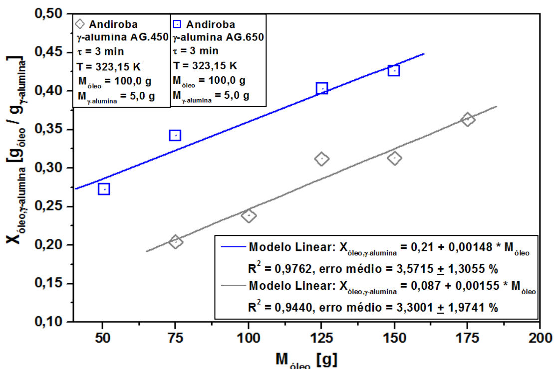
Gráfico 4.8 - Influência da massa de óleo sobre a capacidade de adsorção do óleo de andiroba em \gamma -alumina.
