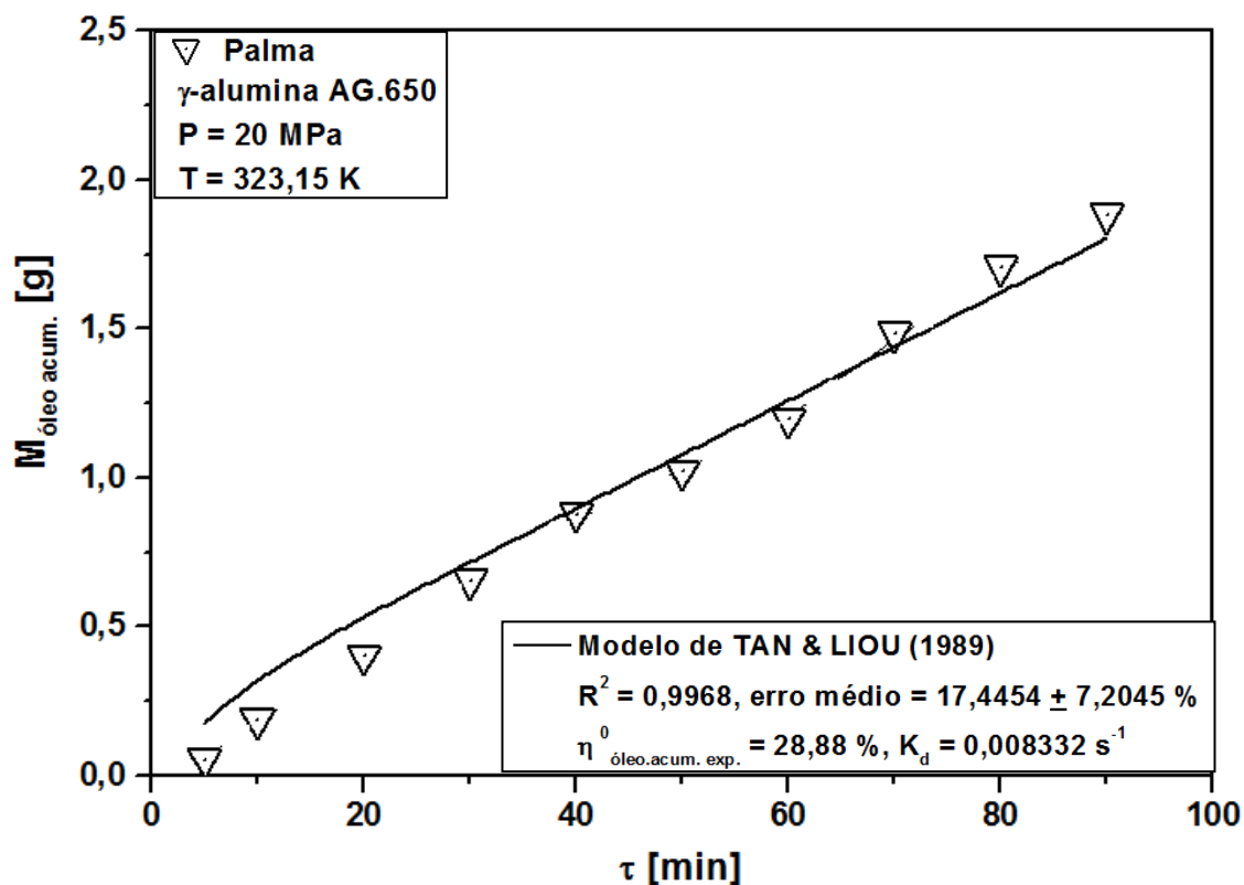
Gráfico 4.21 - Modelagem da curva de dessorção do óleo de palma em \gamma -alumina AG.650 a 20 MPa e 328,15 K utilizando-se o modelo de Tan & Liou.
