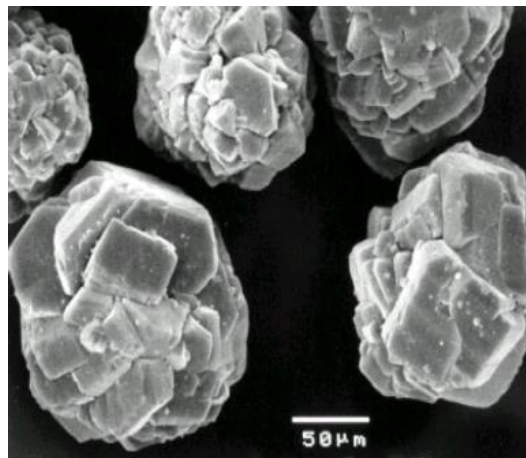
Figura 4.2 - Microscopia eletrônica do adsorvente \gamma –alumina AG.650.
