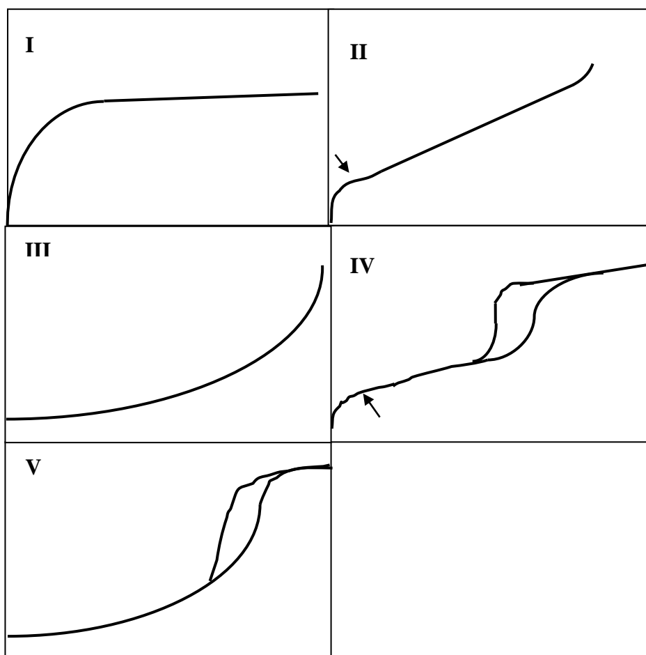
Figura 2.4 - Tipos de isotermas de adsorção (GREGG & SING 1982 apud BRUNAUER et al. 1940).
