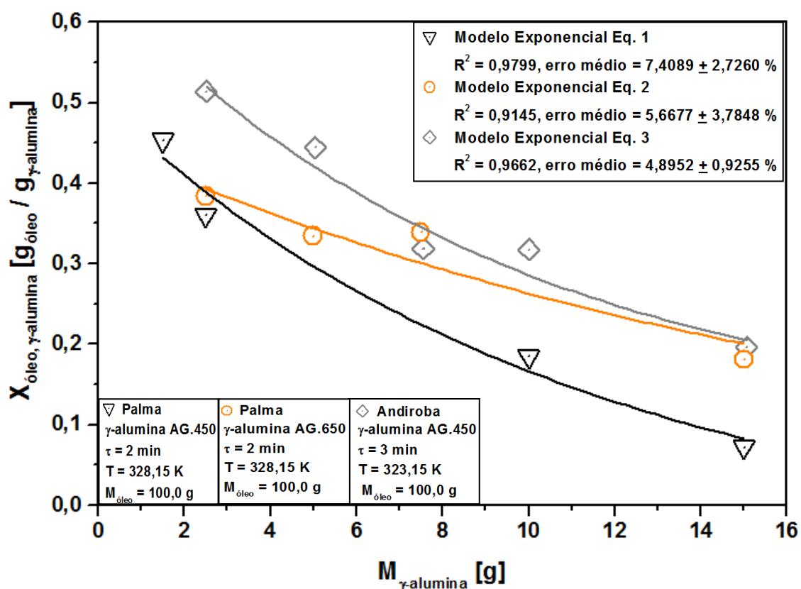
Gráfico 4.2 - Influência da massa de \gamma -alumina sobre a capacidade de adsorção dos óleos de palma e andiroba
