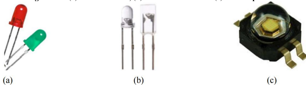
Figura 3.9 - (a) LED indicador, (b) LED de alto brilho e (c) LED de potência.
