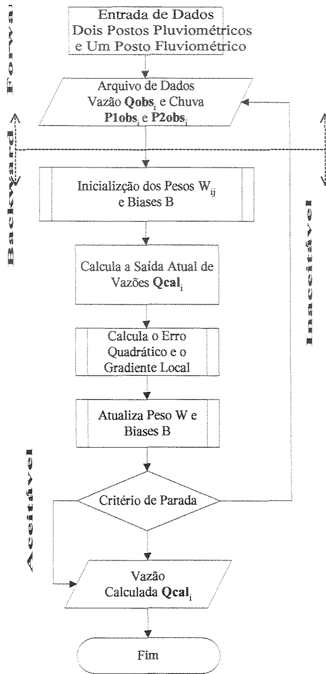
Figura 4.8 – Caso4: Relação Direta Precipitação-Vazão por RNA (dois Postos Pluviométricos)
