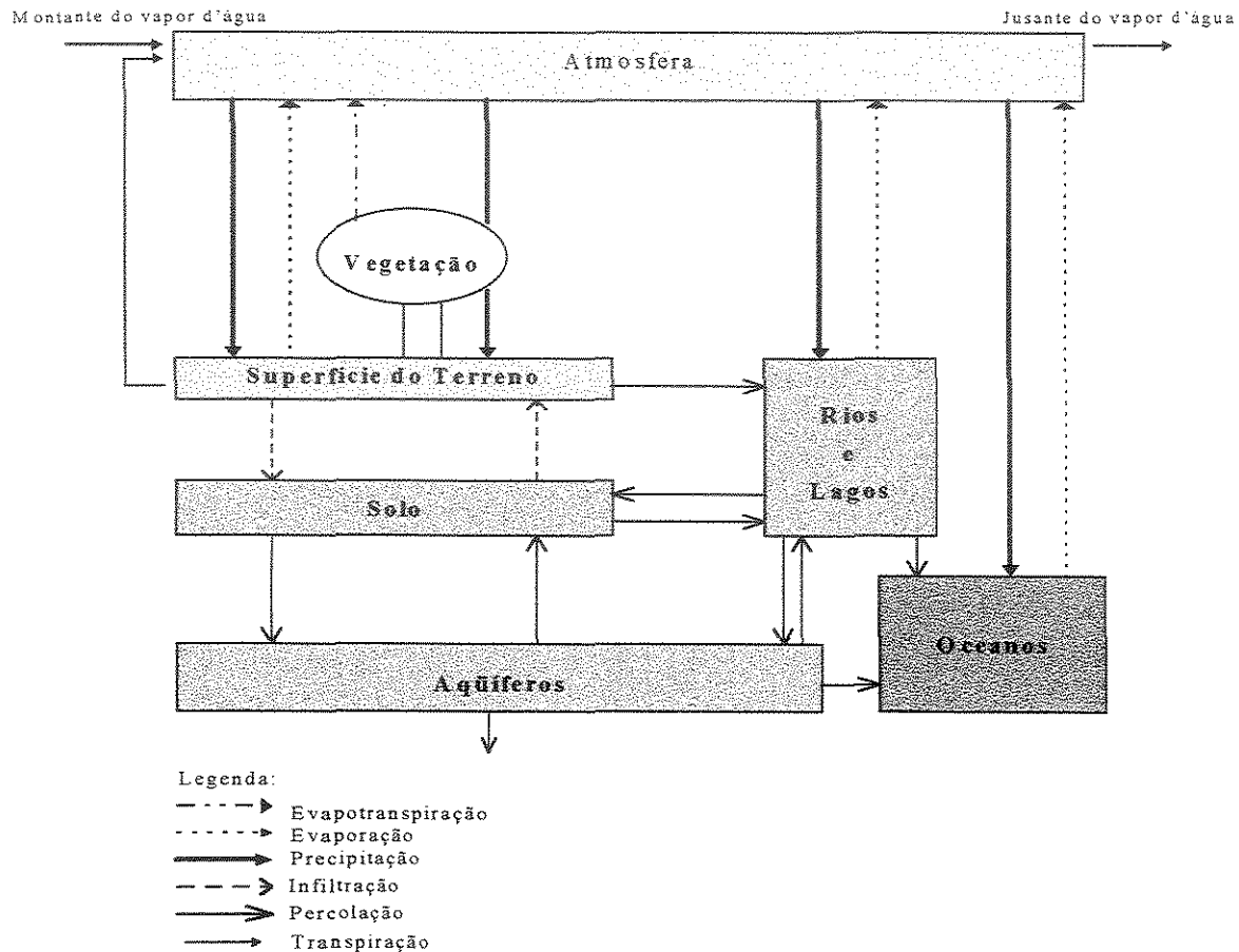
Figura 2.1 - Desenho Esquemático do Ciclo Hidrológico
