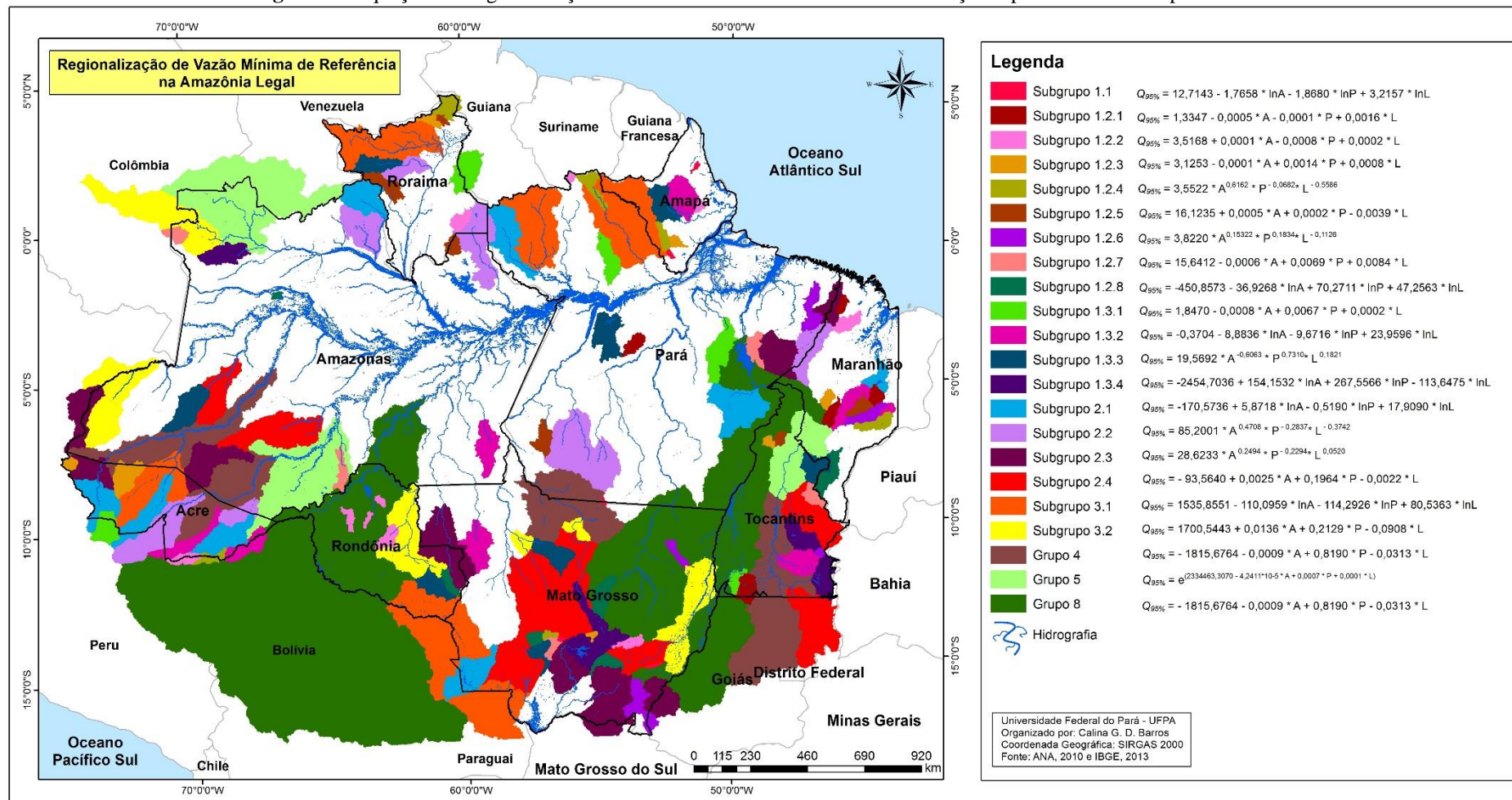
Figura 14. Equações de regionalização da vazão mínima de referência e localização espacial do local de possível uso.
