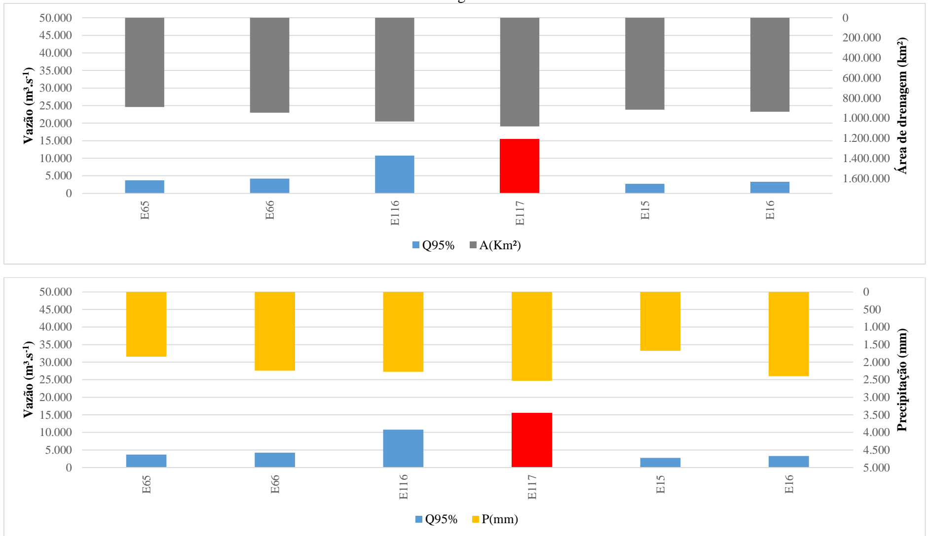
APÊNDICE F – Relação da Q_{95\%} com as variáveis explicativas e o período de dados utilizados, destacando estações retiradas do Grupo Homogêneo 8.
