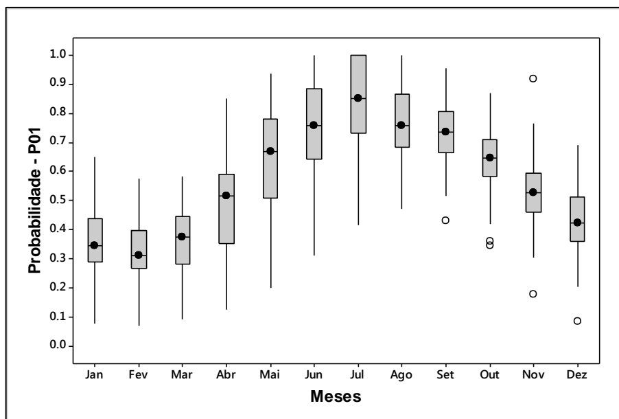
Figura 8 - Box-Plots da probabilidade da sequência de dia atual seco com anterior chuvoso ( P_{01} ) para as 80 estações pluviométricas da BHRT
