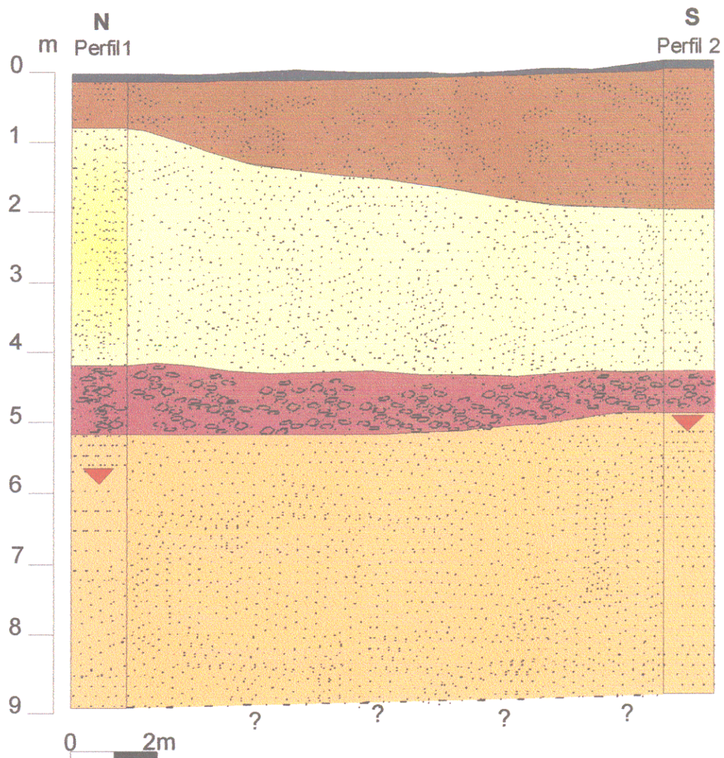
Figura 12 – Seção geológica.
