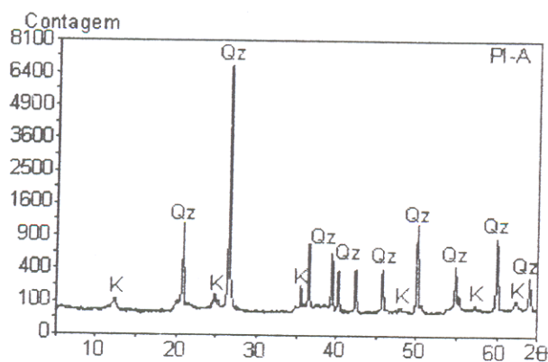
Figura 13 – Difratograma da amostra P1-A
