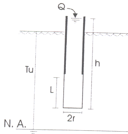
Figura 8: Esquema ilustrando as variáveis envolvidas no cálculo da condutividade hidráulica de solos (extraído de Oliveira & Corrêa Filho 1996).
