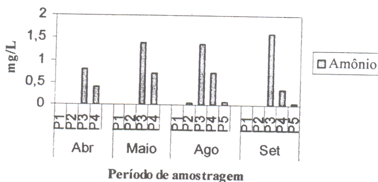
Figura 21 – Variações das concentrações de amônio nos poços de monitoramento no período seco e chuvoso.
