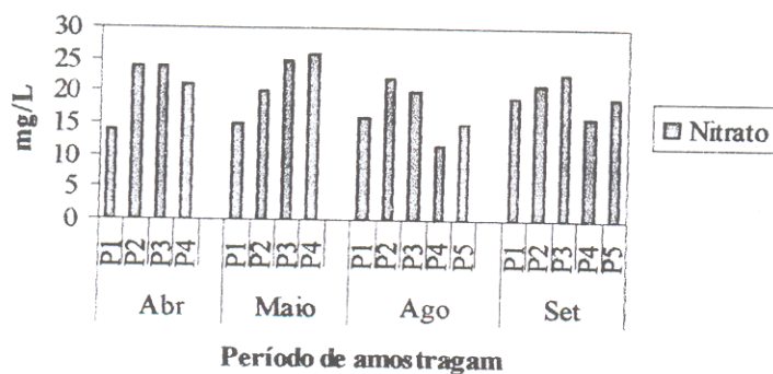
Figura 22 – Gráfico ilustrando o comportamento das concentrações de nitrato nos poços de monitoramento no período seco e chuvoso.
