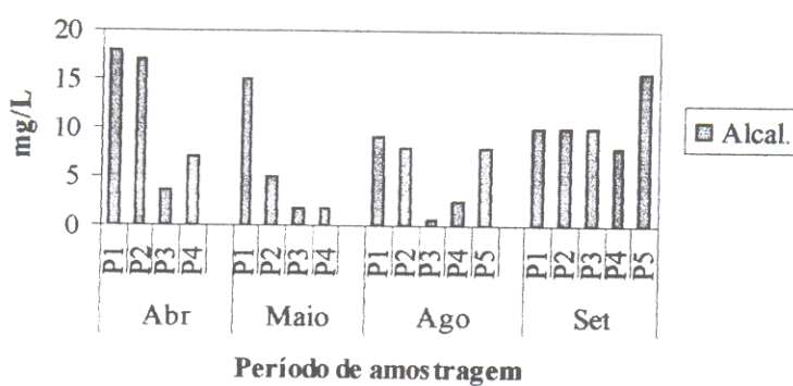
Figura 25 – Variação das concentrações de bicarbonato nos poços de monitoramento no período seco e chuvoso.
