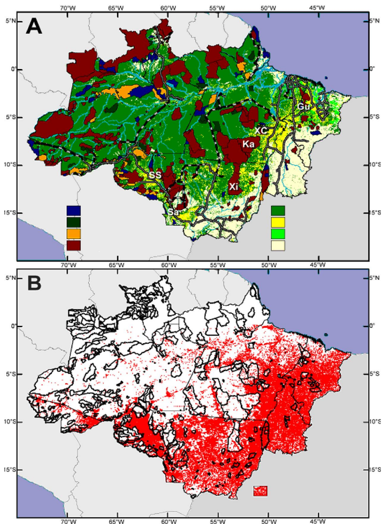
Mapa 27 e 28 - Distribuição do desmatamento e de queimadas (focos de calor) em função dos diferentes tipos de áreas protegidas na Amazônia Legal. Note-se o efeito das terras indígenas como proteros da floresta, sobre a ocorrência de focos de calor. As áreas indígenas conservam a floresta em pé, são barreiras. Fonte: IPAM (2005).
