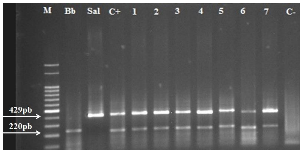
Figura 1. Eletroforese em gel de agarose 1,5% demonstrando os produtos da mPCR-SBb aplicada em amostras comerciais bubalinas identificando contaminação por Salmonella spp. M: marcador de peso molecular de 100pb; Bb: B. bubalis , Sa: Salmonella spp., C+: controle positivo ( Salmonella spp. e B. bubalis ) 1 a 7: Amostras comerciais de cortes cárneos bubalinos comercializados no Pará; C-: controle negativo.
