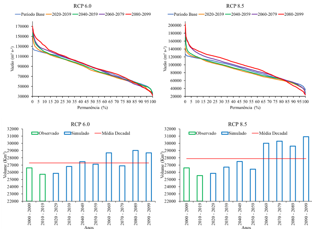
Figura 28 - Projeções WaterGAP2 (MIROC5) de curvas de permanência ( \text{m}^3 \cdot \text{s}^{-1} ) e volume ( \text{km}^3 ) para a estação E4
