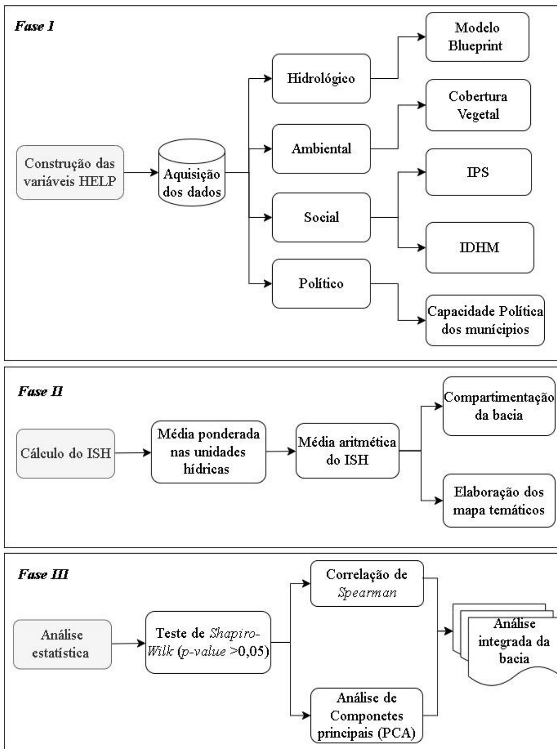
Figura 5- Fluxograma metodológico.
