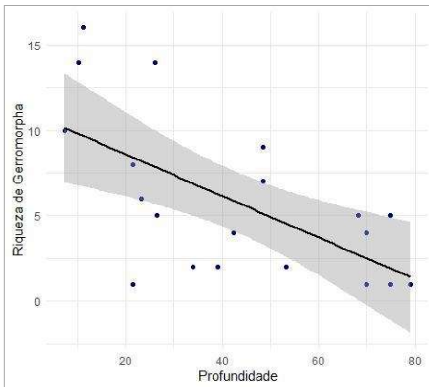
Figura 5 – Relação da variável Profundidade entre a riqueza de espécies da subordem Gerromorpha, nos igarapés amostrados ( r^2 = 0.3556 , p < 0.003269 ).
