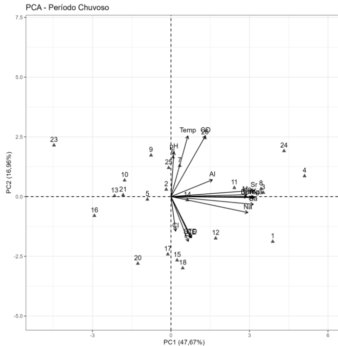
Figura 30 - Plotagem das componentes CP1 e CP2 considerando os parâmetros de qualidade da água para a segunda campanha
