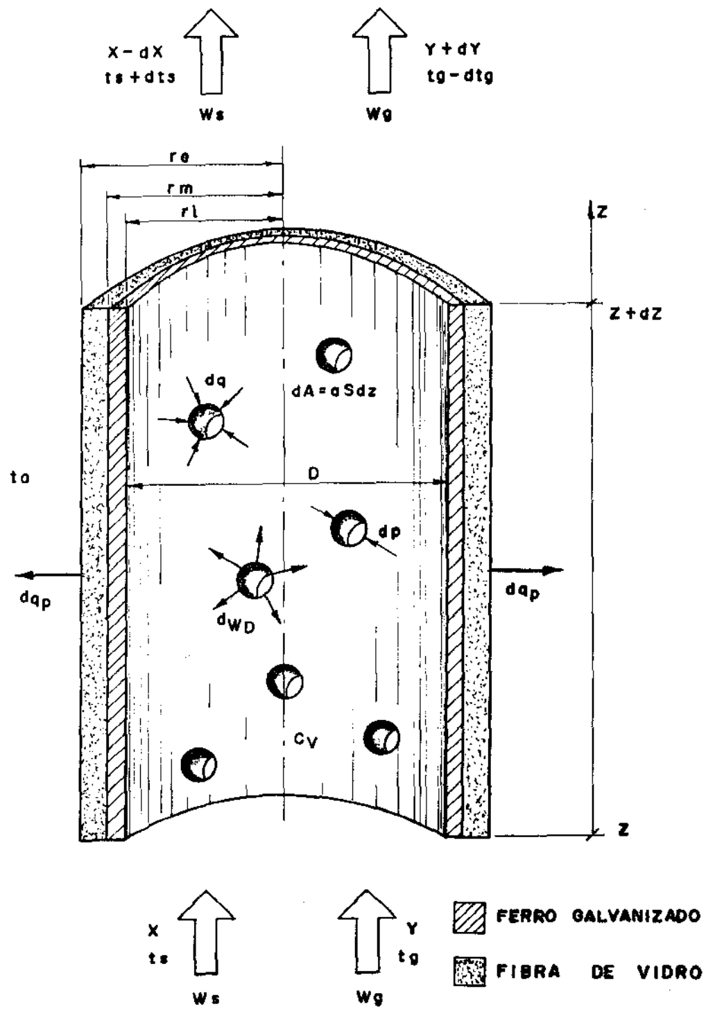
FIGURA 5.1 ESQUEMA DO COMPRIMENTO DIFERENCIAL DO SEGADOR PNEUMÁTICO
