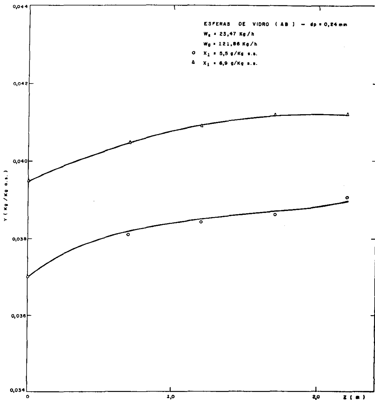
FIGURA 6.1 — PERFIL DE UNIDADE DO AR ( INFLUÊNCIA DA UNIDADE DE ENTRADA DOS SÓLIDOS )
