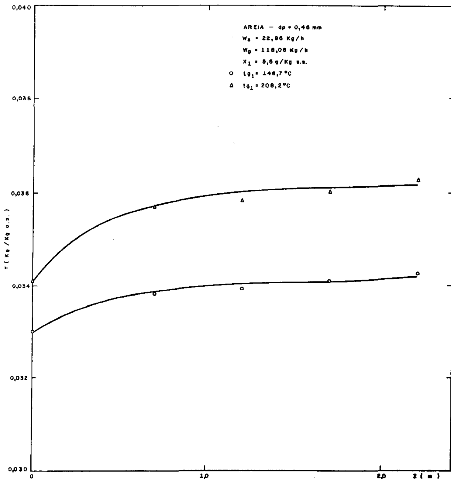
FIGURA 6.5 — PERFIL DE UNIDADE DO AR (INFLUÊNCIA DA TEMPERATURA DE ENTRADA DO AR)
