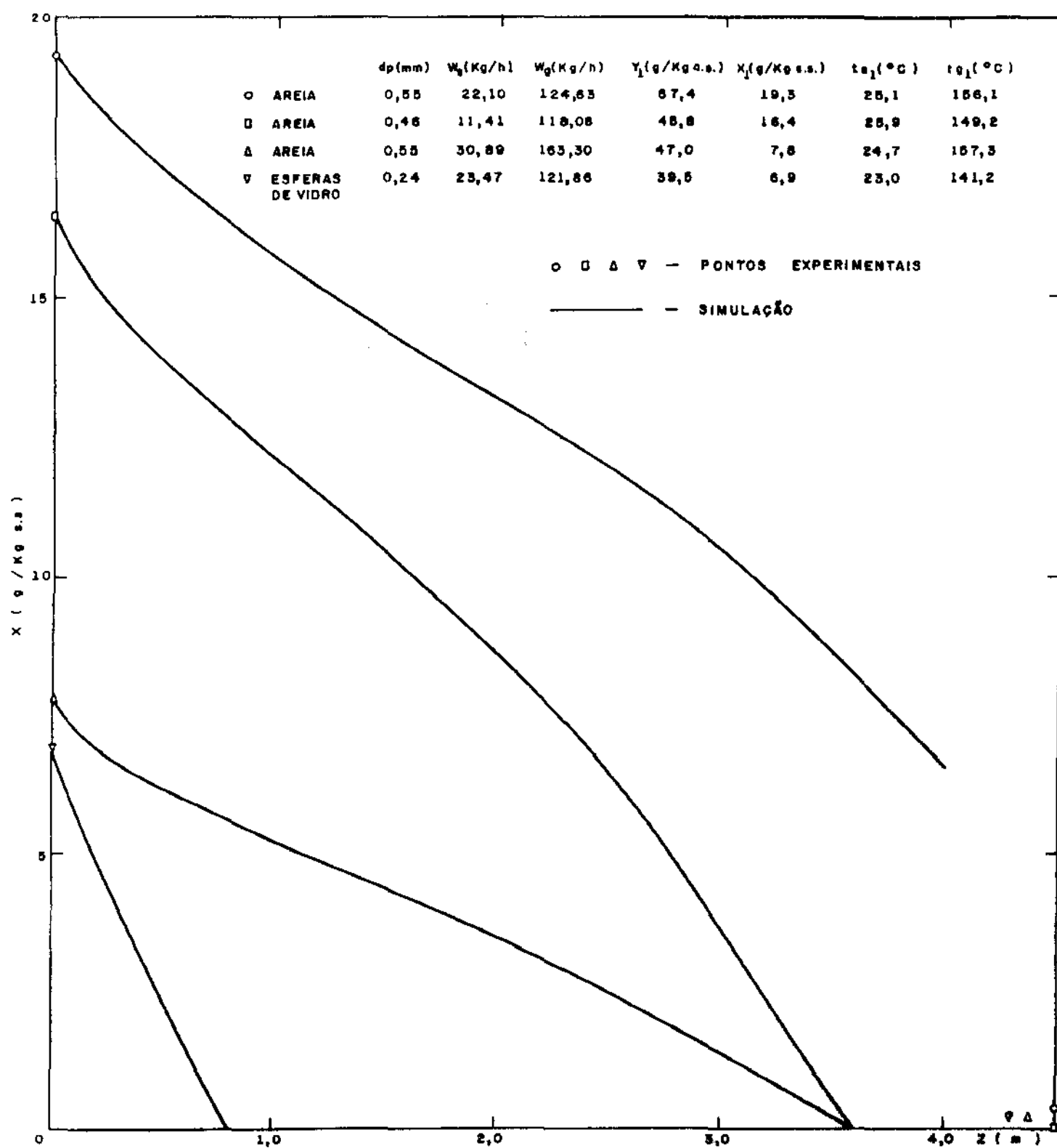
FIGURA 6.14 — PERFIS DE CONTEÚDO DE UNIDADE DOS SÓLIDOS
