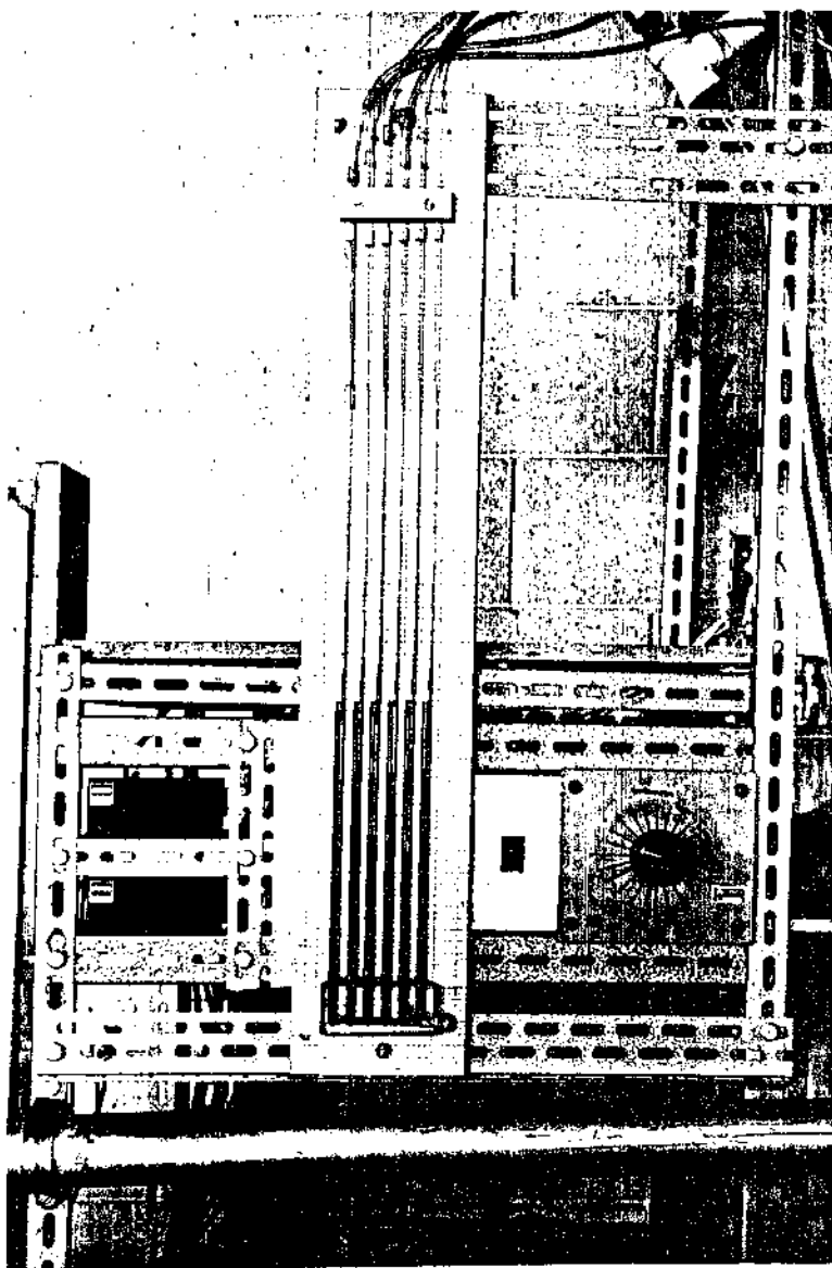
Figura 4.8 - Painel de Medição
