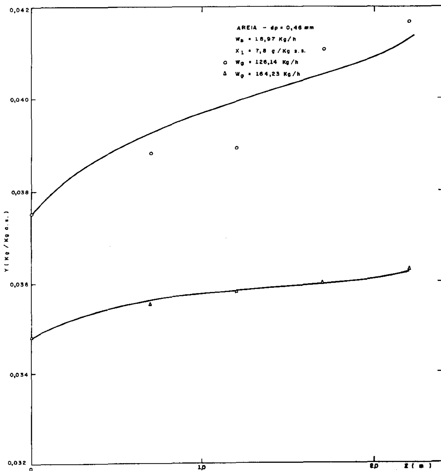
FIGURA 6.9 - PERFIL DE UNIDADE DO AR ( INFLUÊNCIA DA VAZÃO DO AR )
