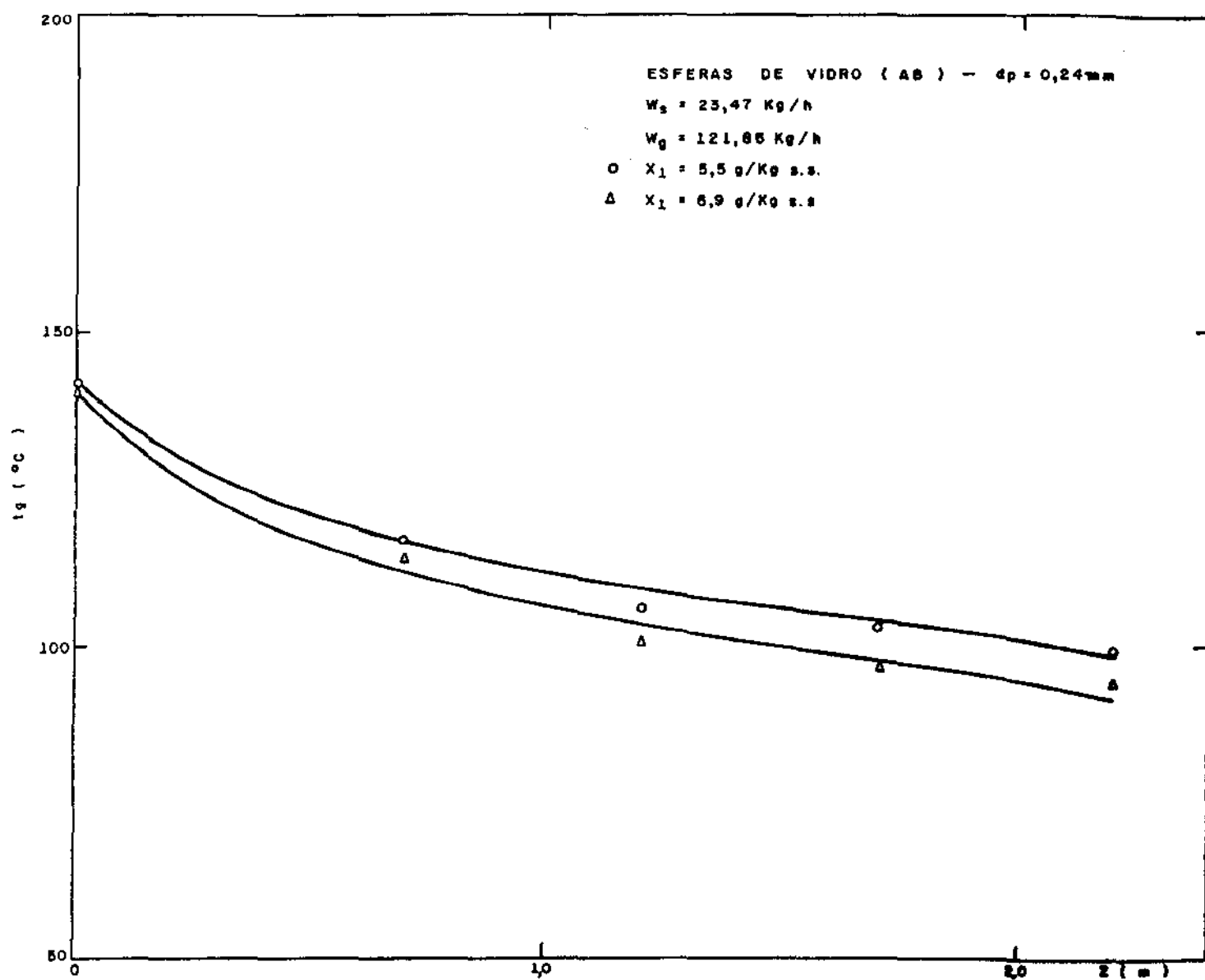
FIGURA 6.2 — PERFIL DE TEMPERATURA DO AR ( INFLUÊNCIA DA UNIDADE DE ENTRADA DOS SÓLIDOS )
